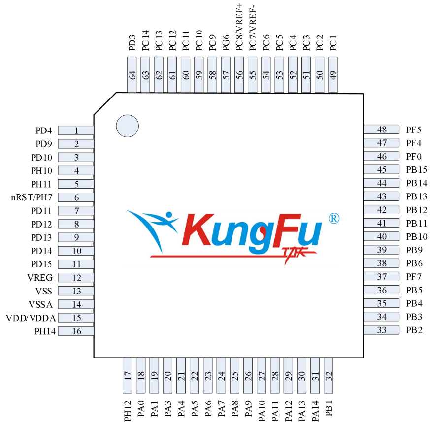
图 2-7 LQFP64
