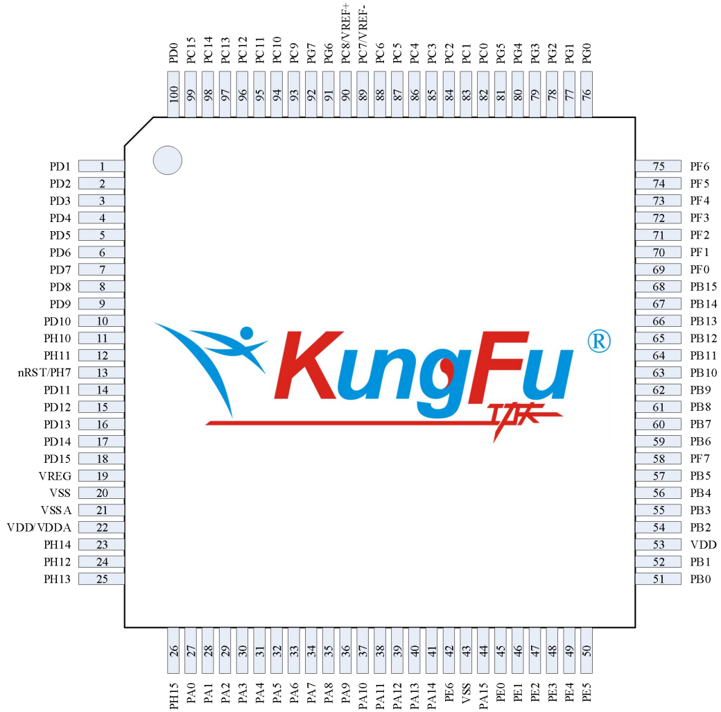
图 2-8 LQFP100
