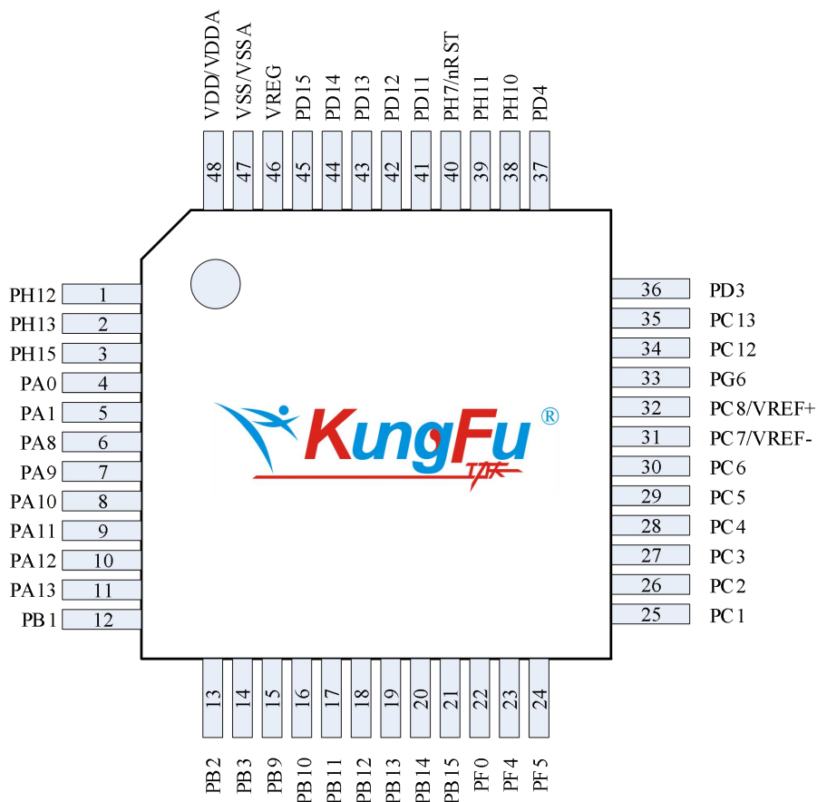
图 2-6 LQFP48
