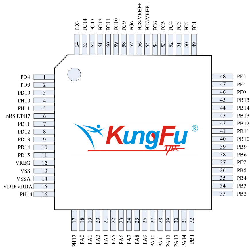
图 2-7 LQFP64
