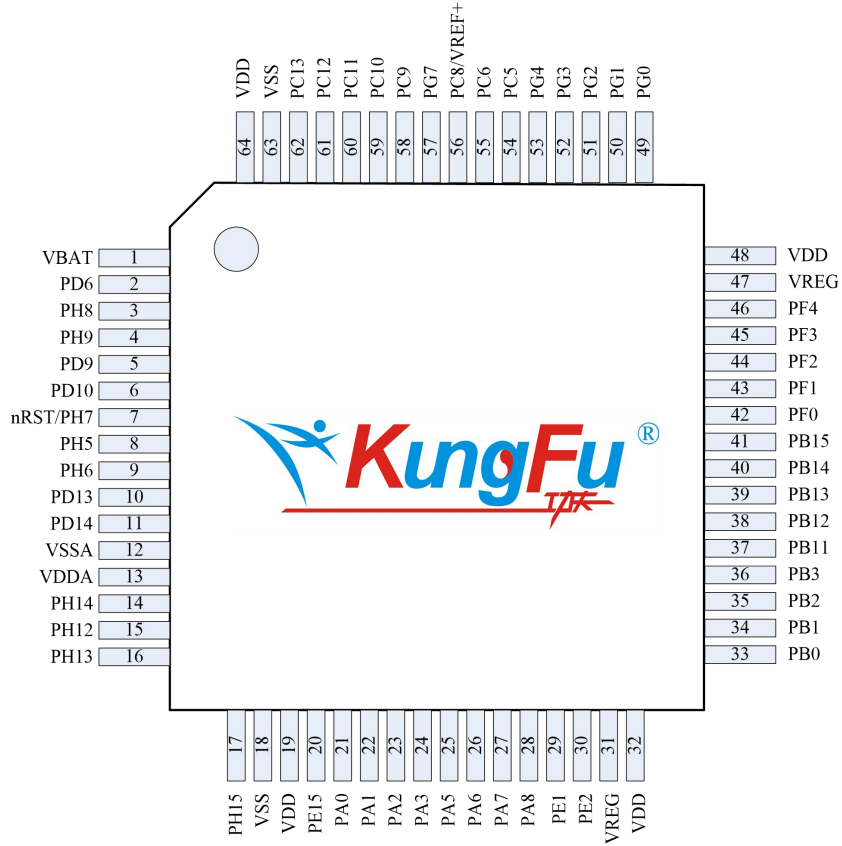
图 2- 5 LQFP64
