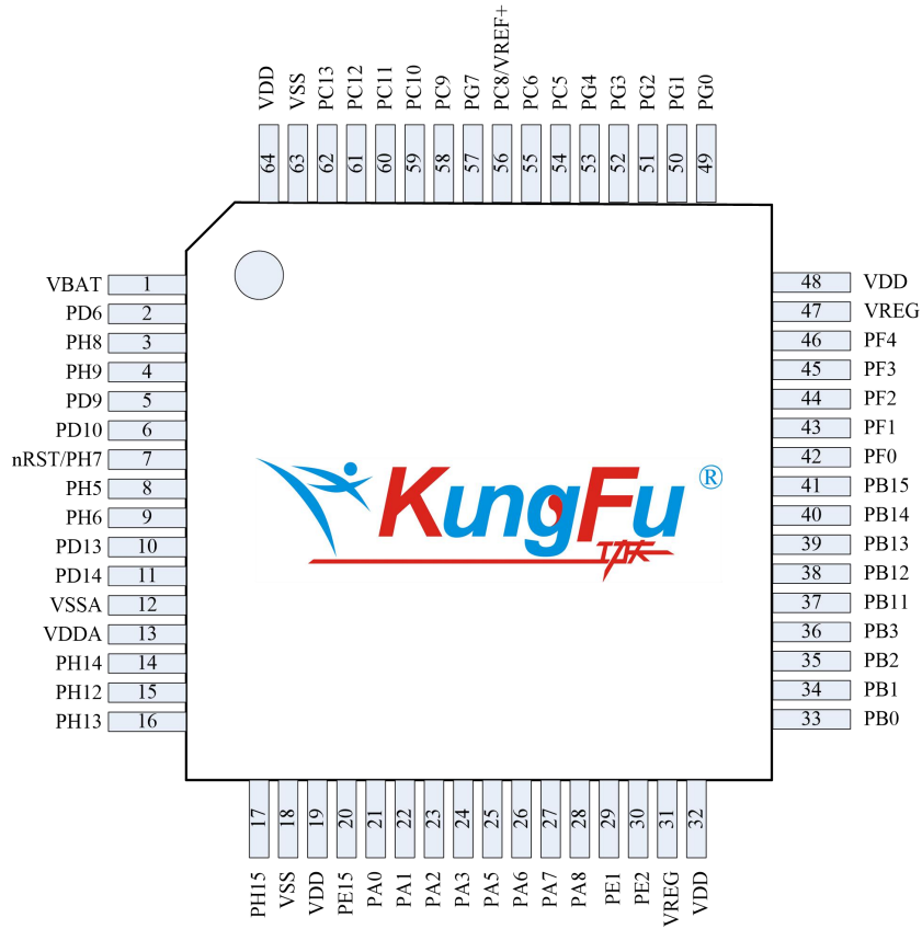
图 2-5 LQFP64
