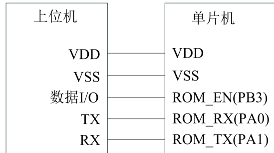
图 2-1 ISP 模式编程接口
