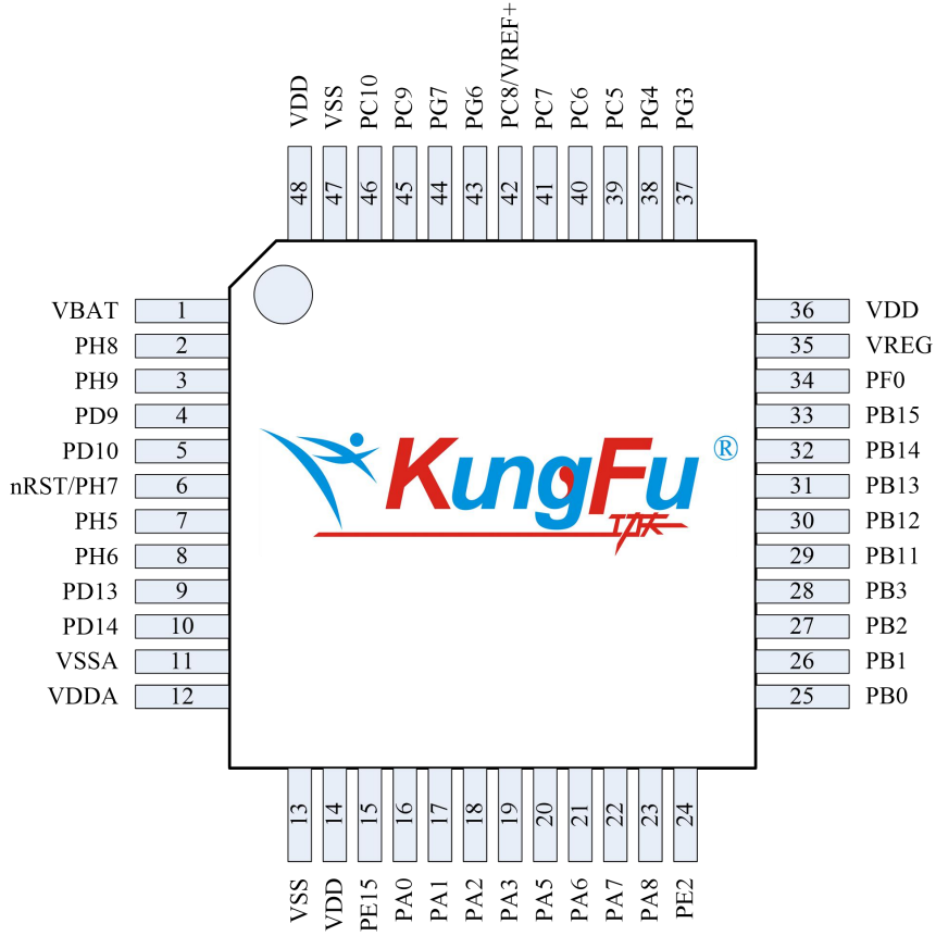
图 2-6 LQFP48
