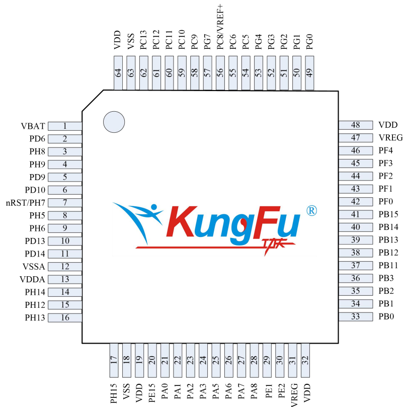
图 2-4 LQFP64
