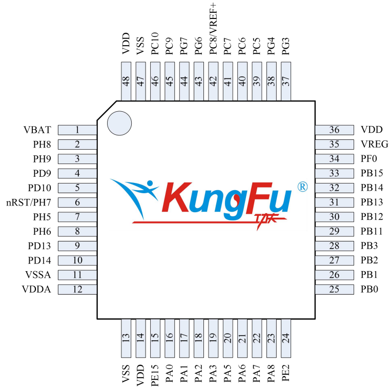
图 2-5 LQFP48
