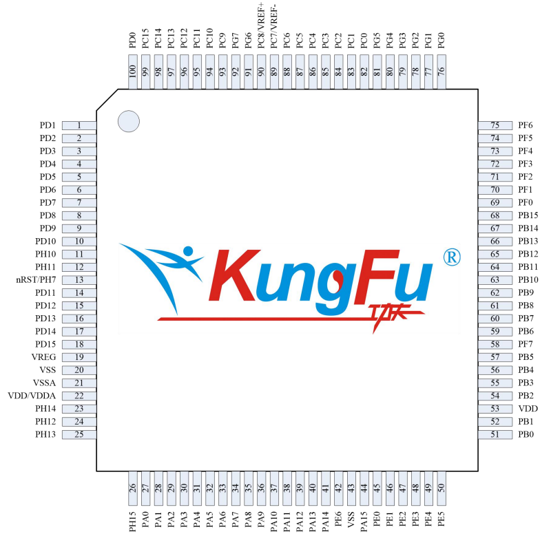
图 2-8 LQFP100
