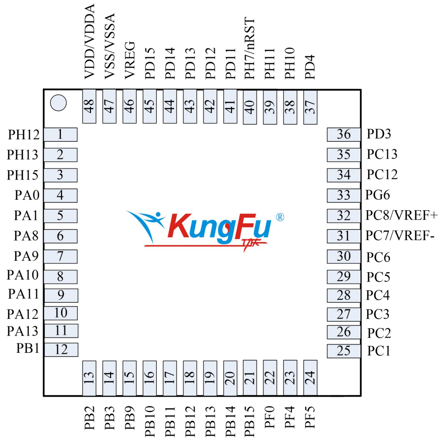
图 2-5 QFN48
