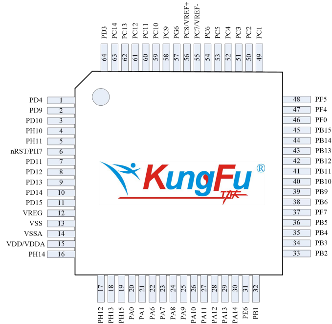
图 2-7 LQFP64
