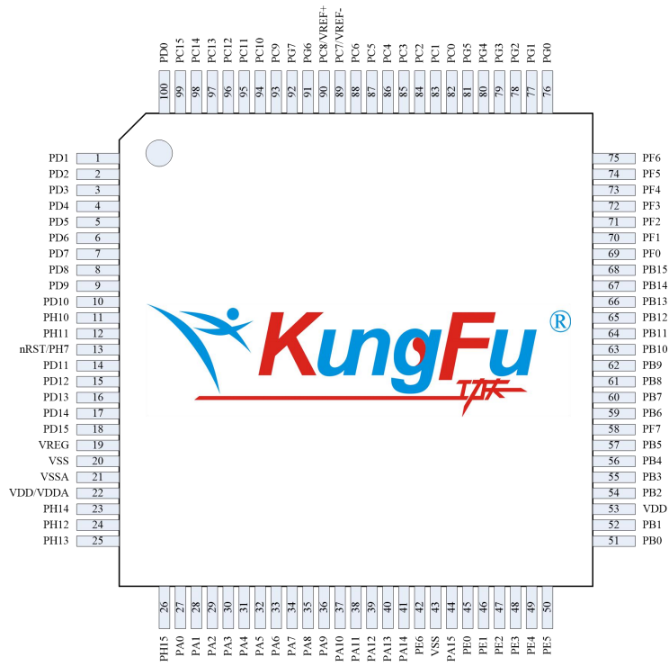
图 2- 8 LQFP100
