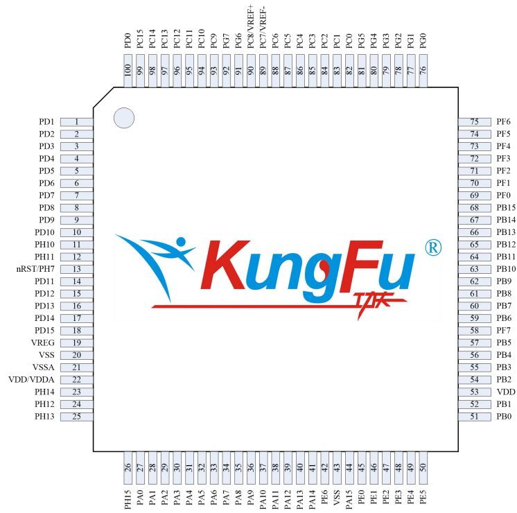
图 2-8 LQFP100
