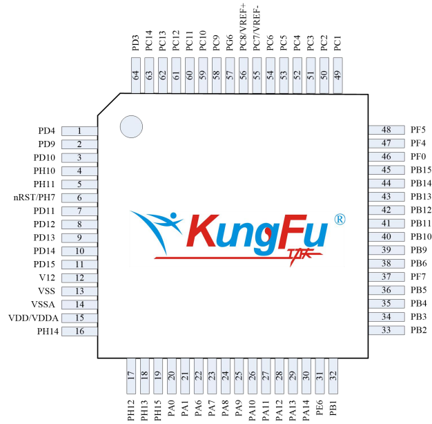
图 2-7 LQFP64
