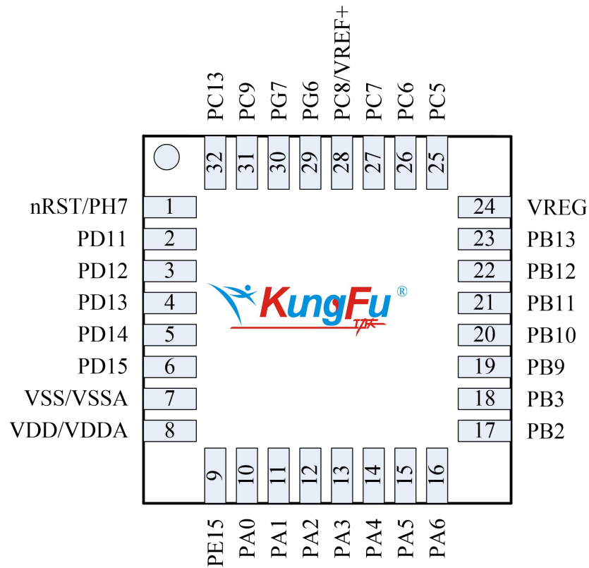
图 2-4 QFN32
