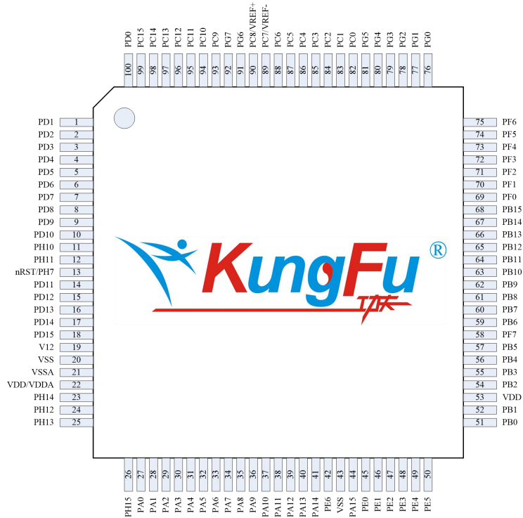
图 2-8 LQFP100
