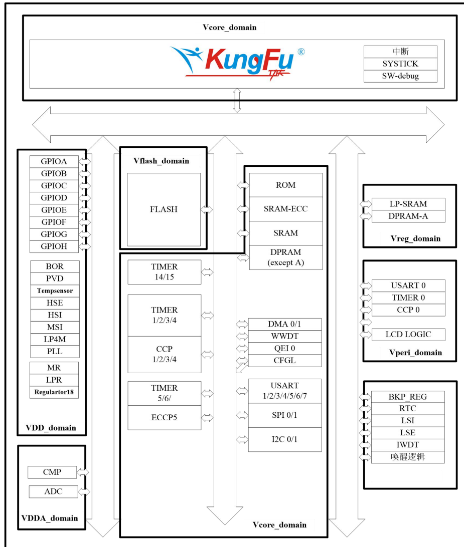
图 2-3 系统结构框图
