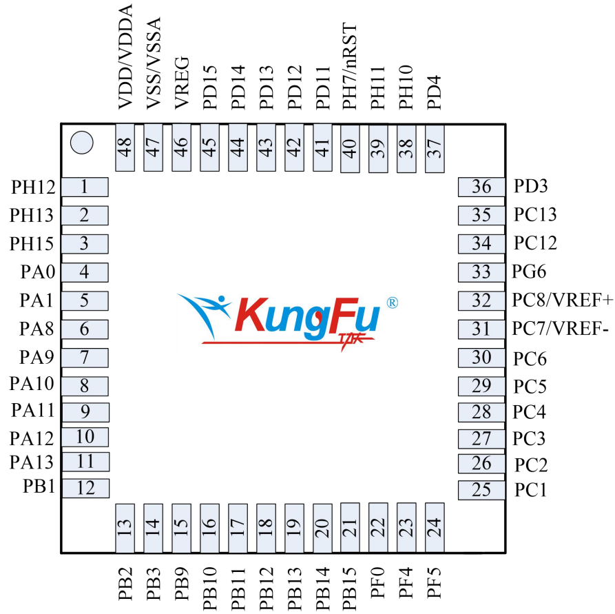
图 2-5 QFN48
