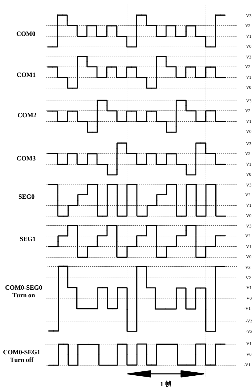
图 17.13 在 1/4 复用、1/3 偏置驱动时的 A 型波形
