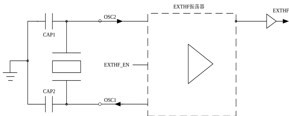
图 3.3 外部高频振荡器原理图
