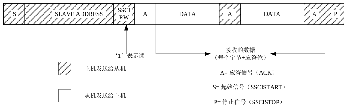
图 16.15 I2C 协议典型读数据帧格式
