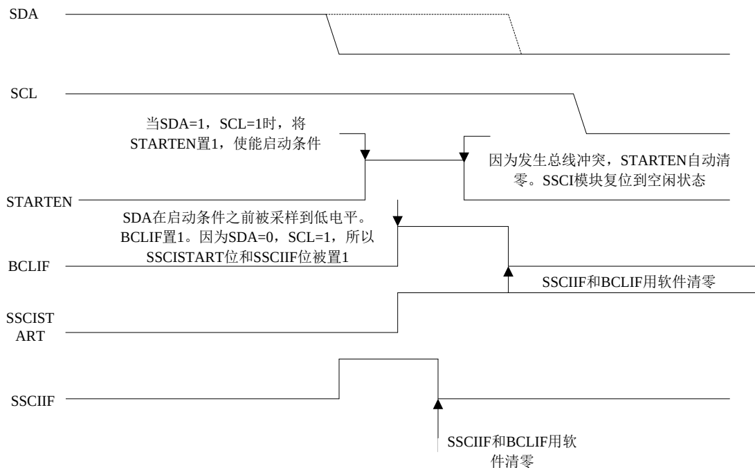
图 16.21 启动条件期间的总线冲突（仅 SDA）
