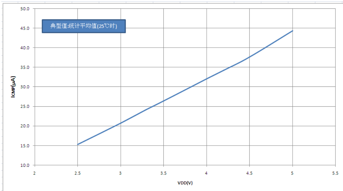
图 26.8:比较器电流 I_{CMP} — V_{DD} 关系曲线图（使能一路比较器）
