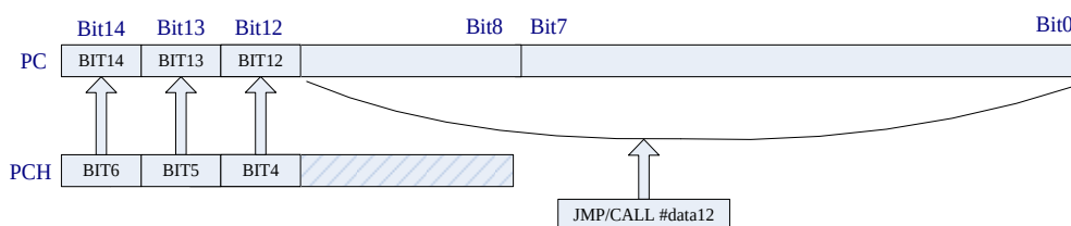
图 4.5 执行 JMP/CALL 指令时 PC 的变化图
