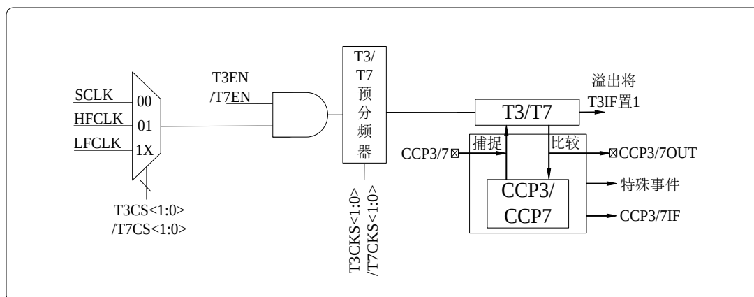
图 8.3 T3/T7 原理框图
