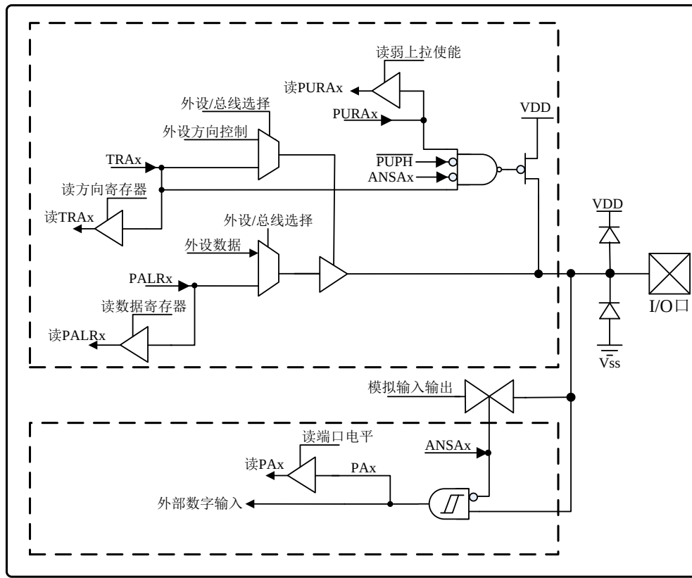
图 2.13 PA 口引脚原理功能框图
