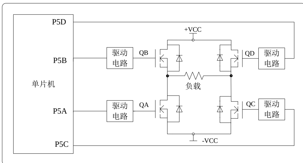
图 13.13 全桥输出模式应用电路示例
