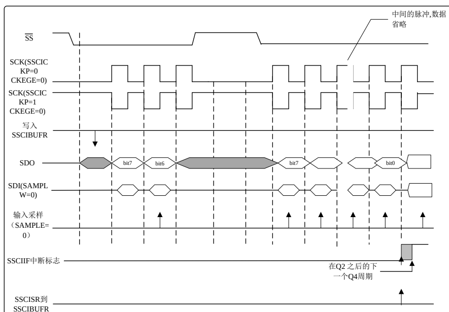
图 16.31 从动时序图
