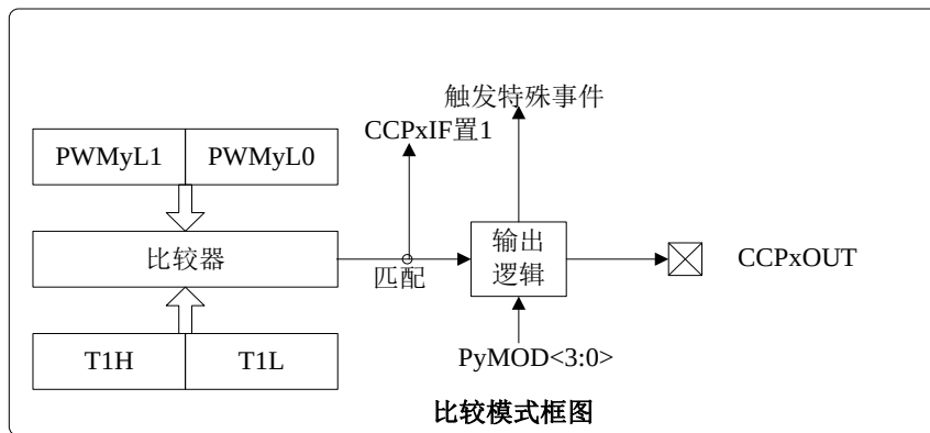
图 12.2 比较模式原理框图
