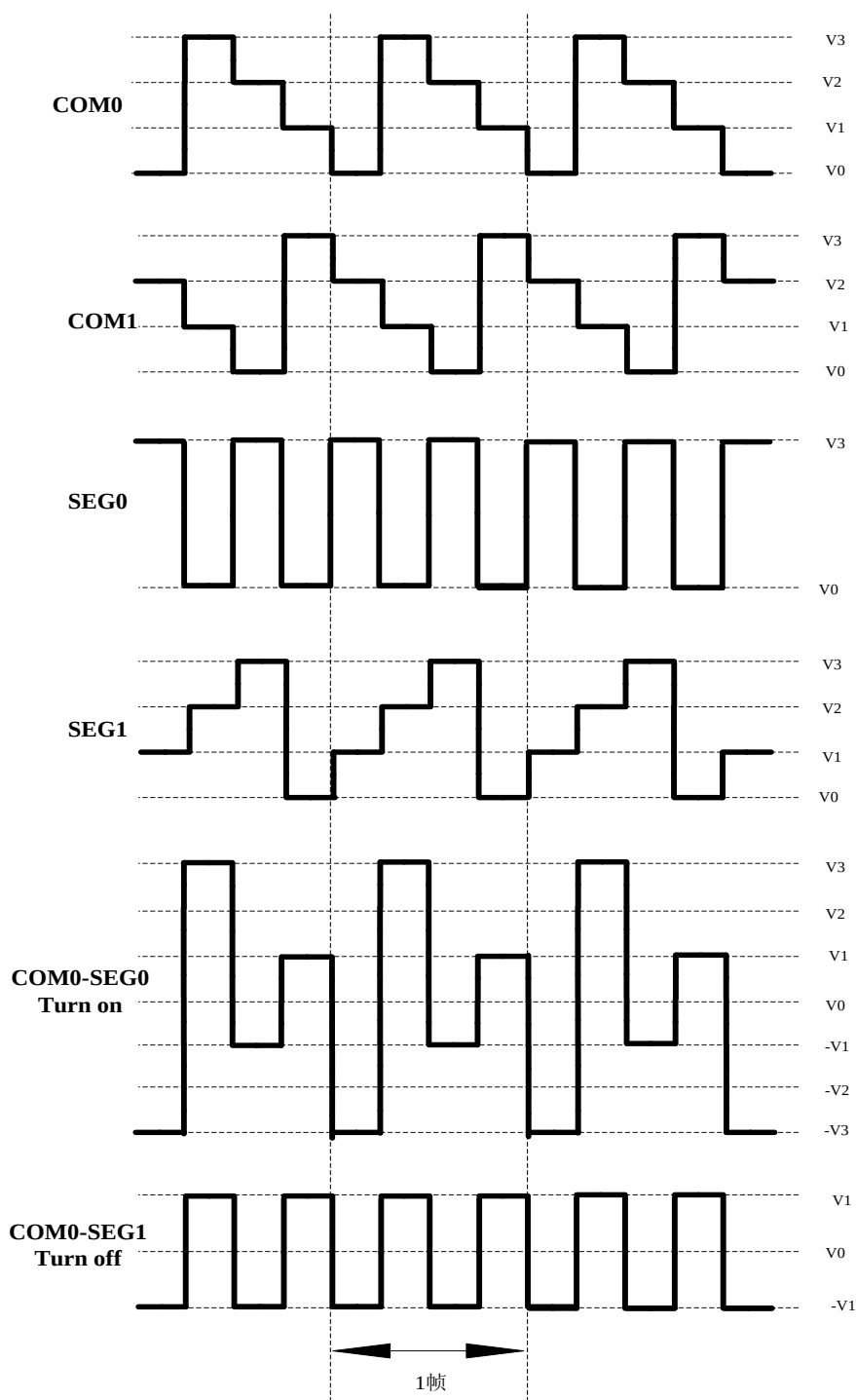
图 17.7 在 1/2 复用，1/3 偏置驱动时的 A 型波形
