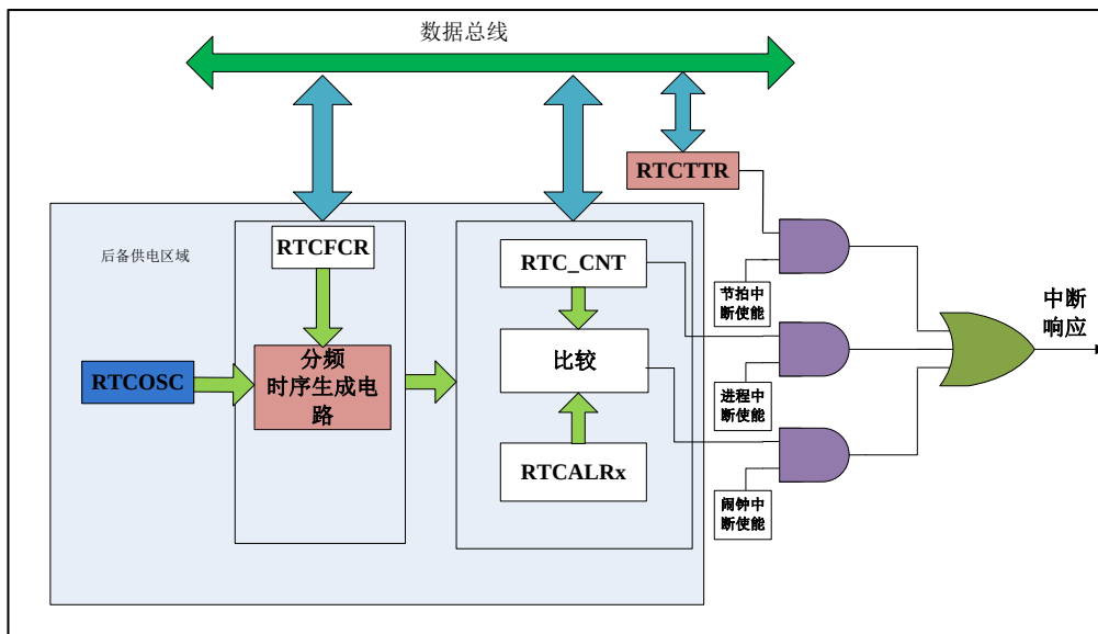
图 20.1 RTC 原理框图
