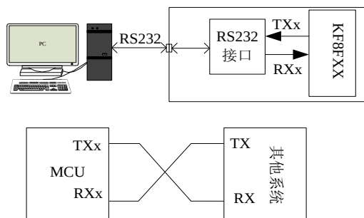
图 15.8 串口通信原理框图
