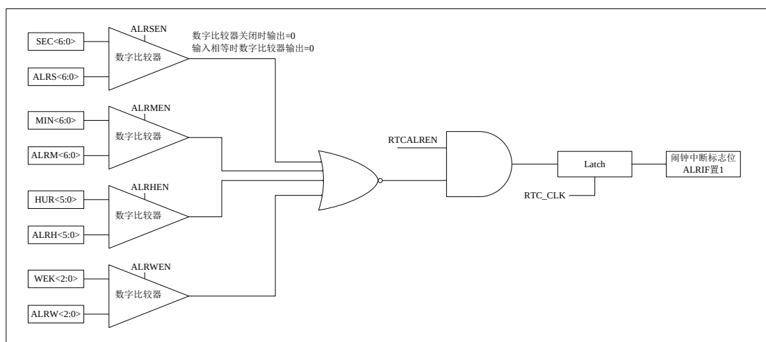
图 20.2 RTC 闹钟功能原理框图
