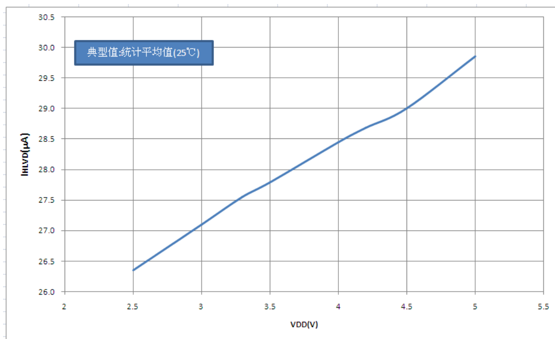
图 26.10:欠压复位电流 I_{HLVD} — V_{DD} 关系曲线图
