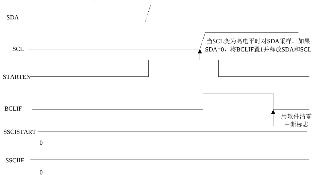
图 16.24 重复启动条件期间的总线冲突（情形 1）
