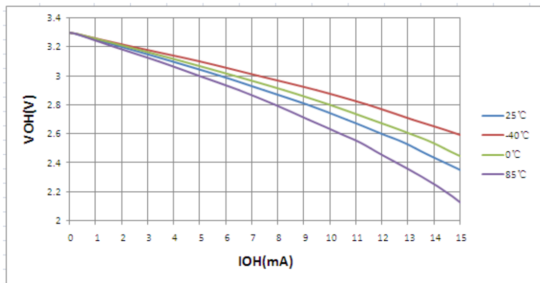
图 26.14:不同温度时 V_{OH} — I_{OH} 关系曲线图 ( V_{DD} = 3.0V )
