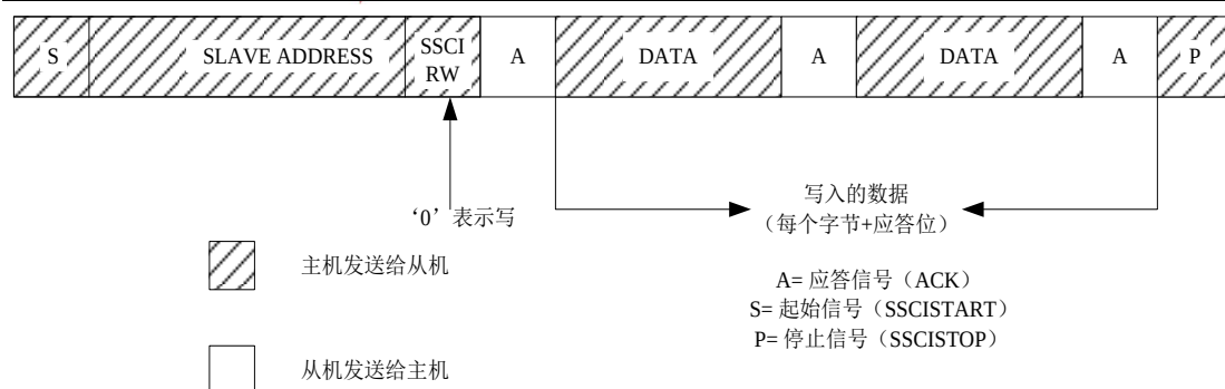
图 16.13 I2C 协议典型写数据帧格式
