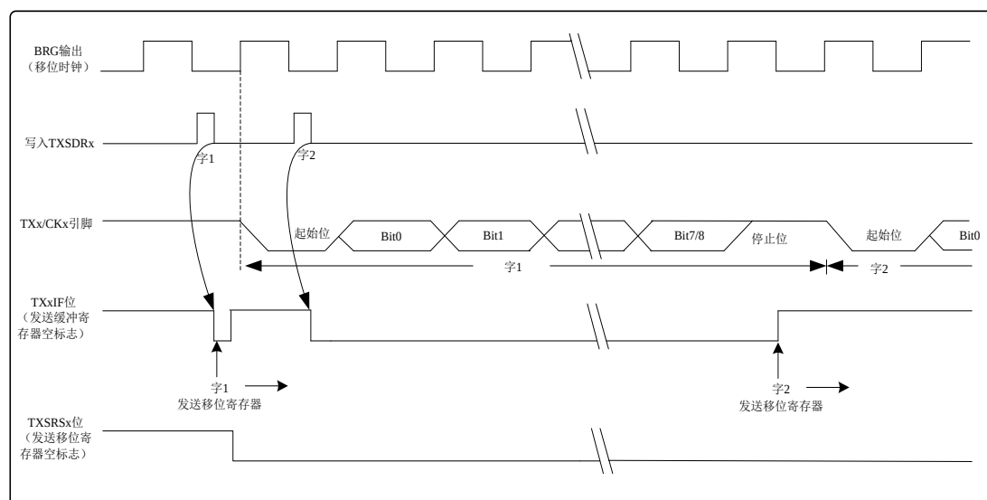
图 15.10 全双工异步发送（一字符接一字符）
