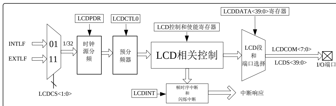
图 17.1 LCD 显示框图
