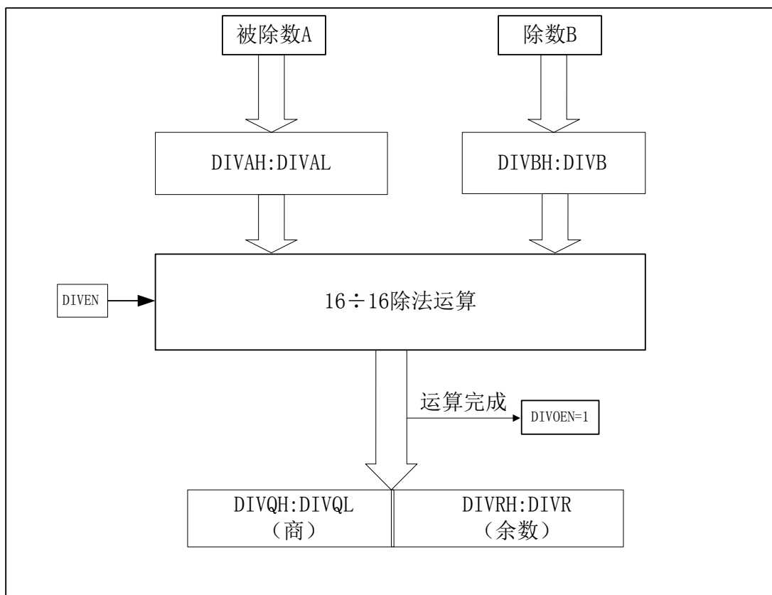
图 19.1 硬件除法器原理框图
