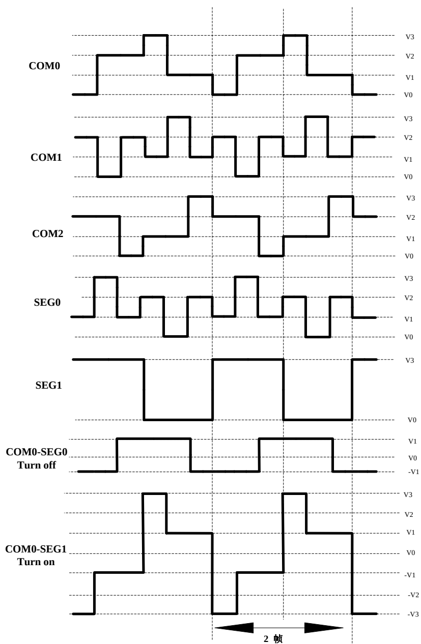
图 17.12 在 1/3 复用、1/3 偏置驱动时的 B 型波形
