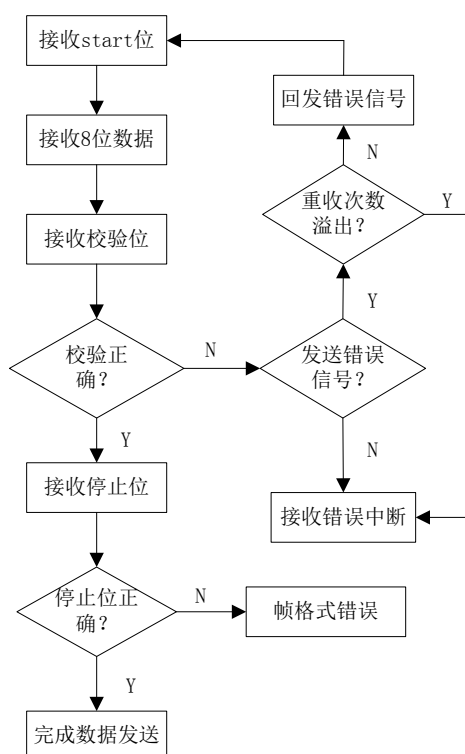
图 15.20 数据接收流程
