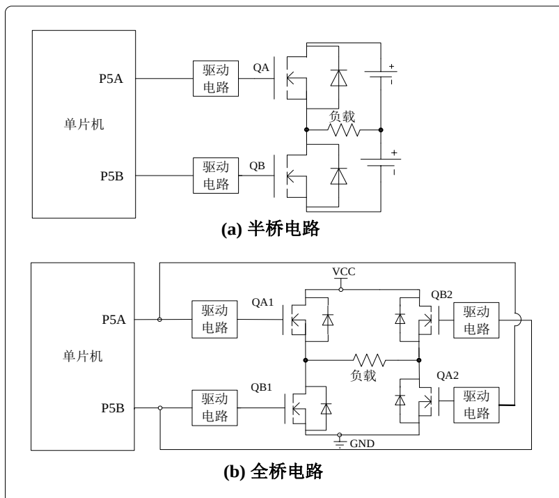
图 13.9 半桥输出模式应用举例
