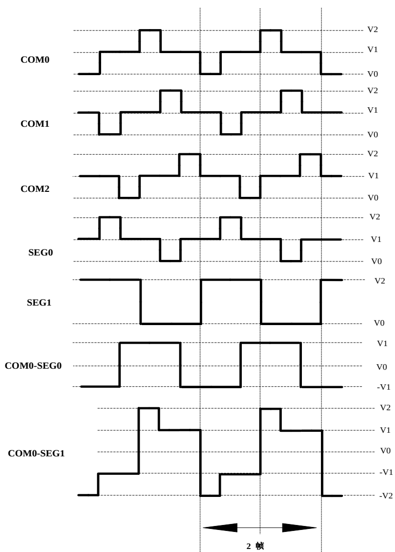
图 17.10 在 1/3 复用、1/2 偏置驱动时的 B 型波形
