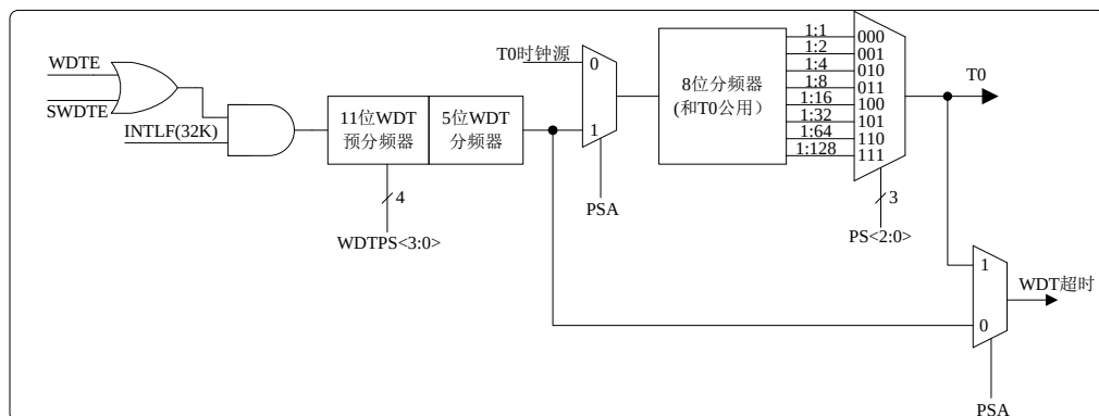
图 23.1 看门狗定时器框图
