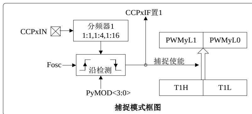
图 12.1 捕捉模式原理框图
