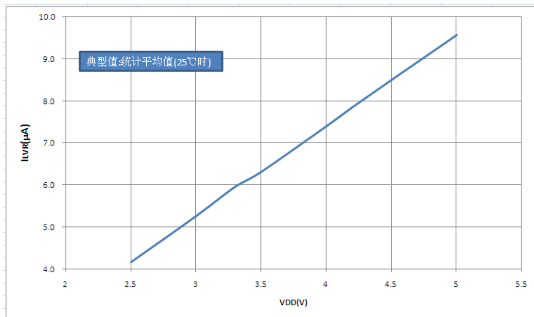
图 26.9:欠压复位电流 I_{LVR} — V_{DD} 关系曲线图
