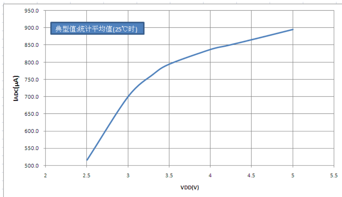
图 26.11: 欠压复位电流 I_{ADC} — V_{DD} 关系曲线图
