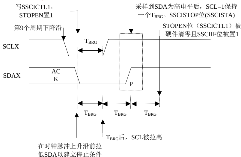
图 16.18 停止条件接收或发送模式
