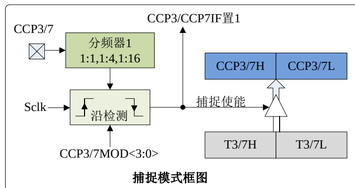
图 8.4 捕捉模式原理框图
