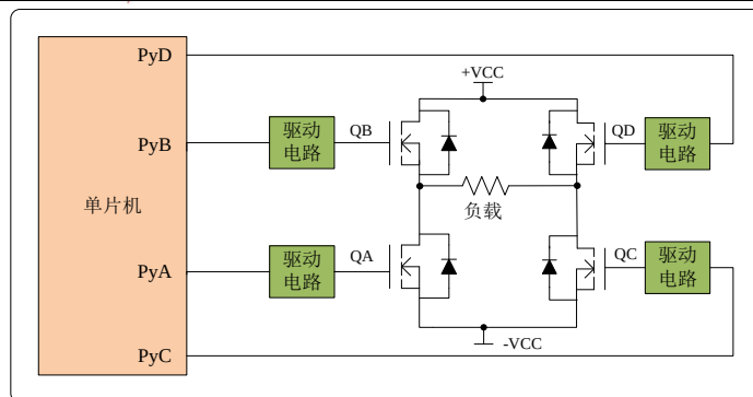
图 12.11 全桥输出模式应用电路示例
