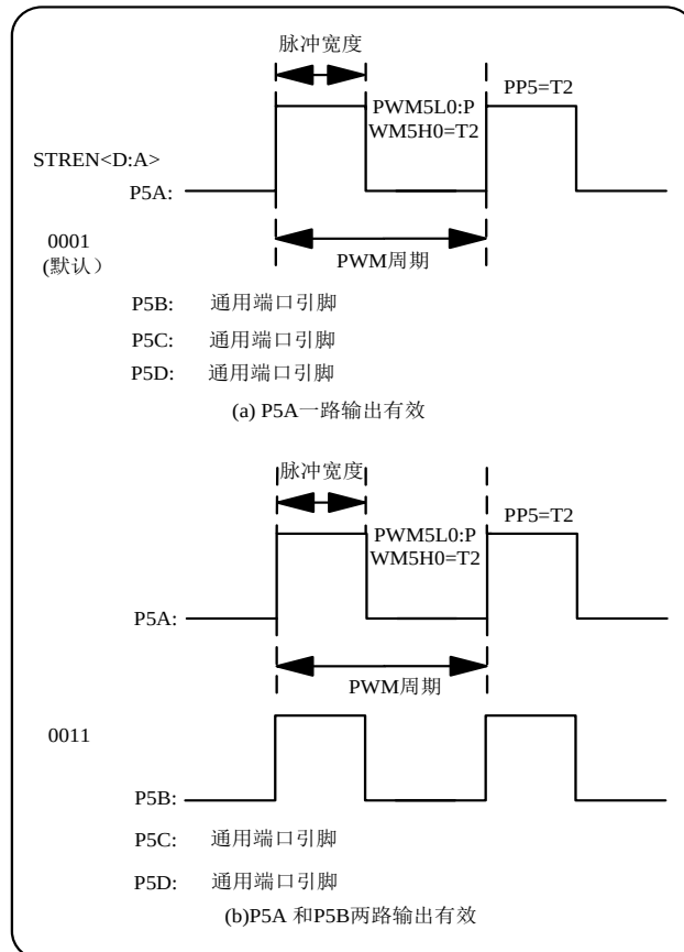
图 13.6 PWM5 的输出示例
