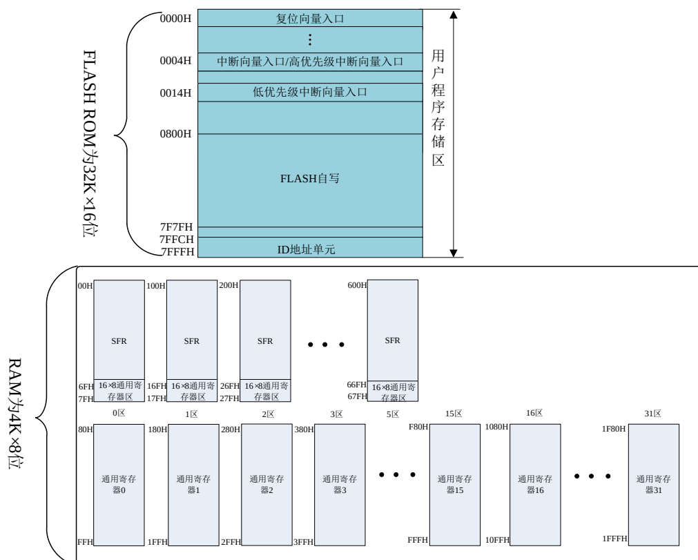
图 4.1 存储器组织图
