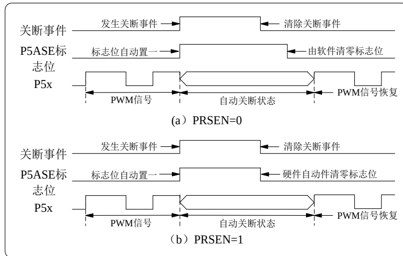
图 13.17 自动重启和软件重启 PWM 示例
