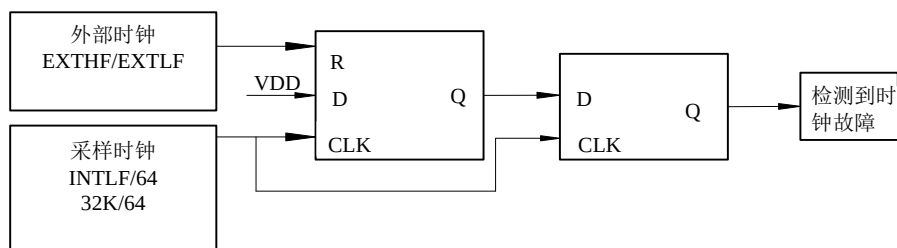
图 3.9 时钟故障检测原理图
