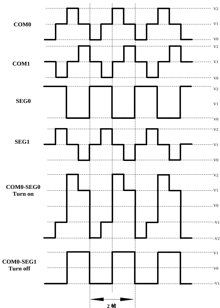
图 17.6 在 1/2 复用、1/2 偏置驱动时的 B 型波形
