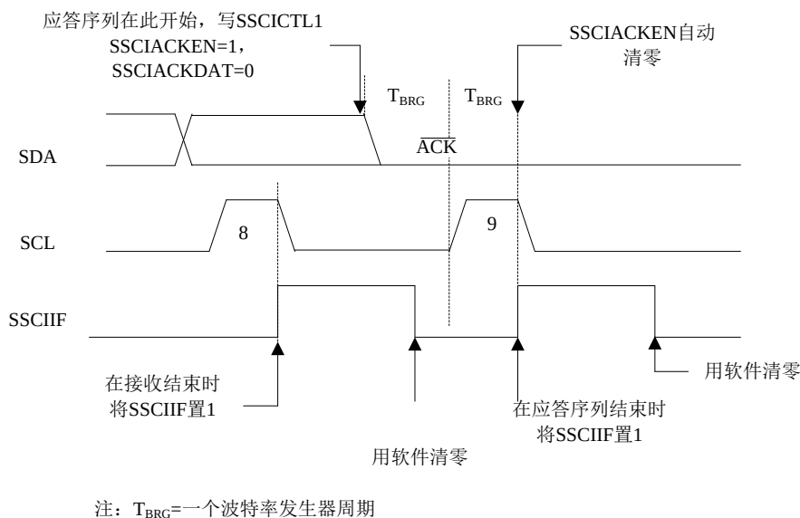
图 16.17 应答序列时序波形
