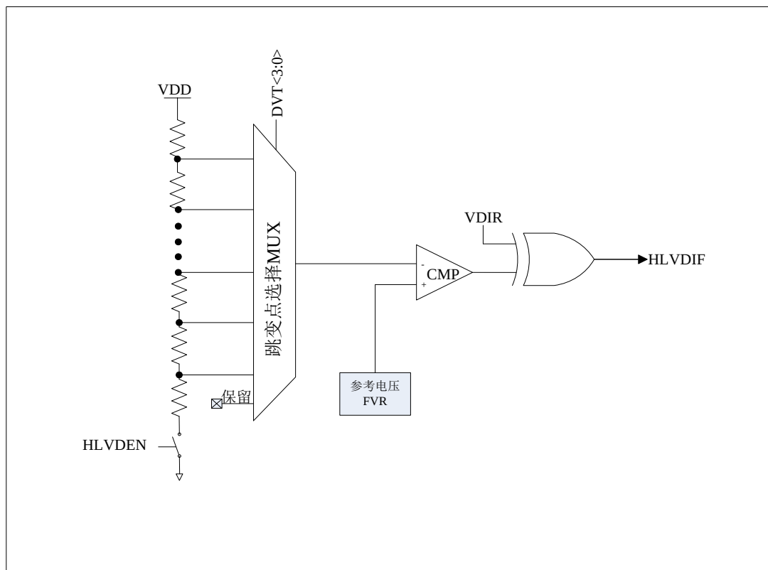
图 22.1 高低压检测原理图
