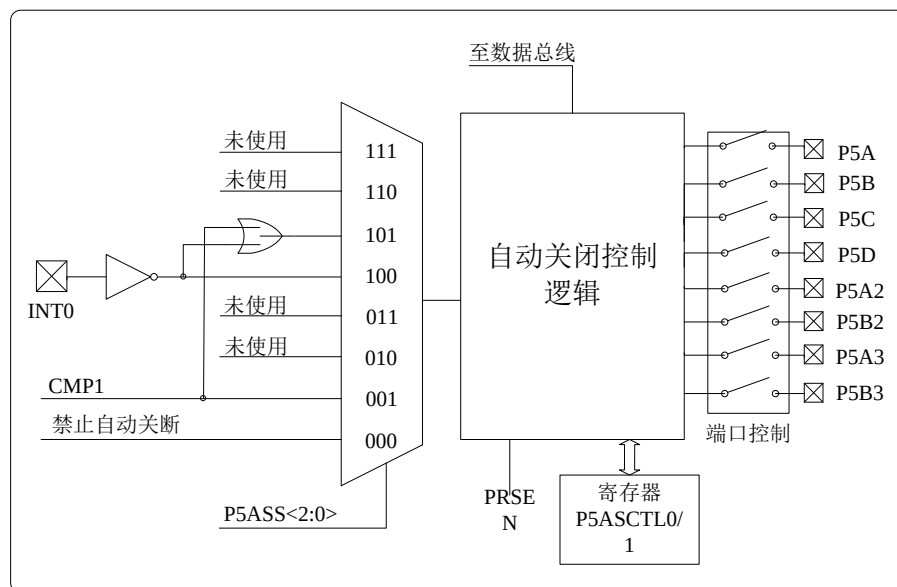
图 13.16 自动关断模式原理框图
