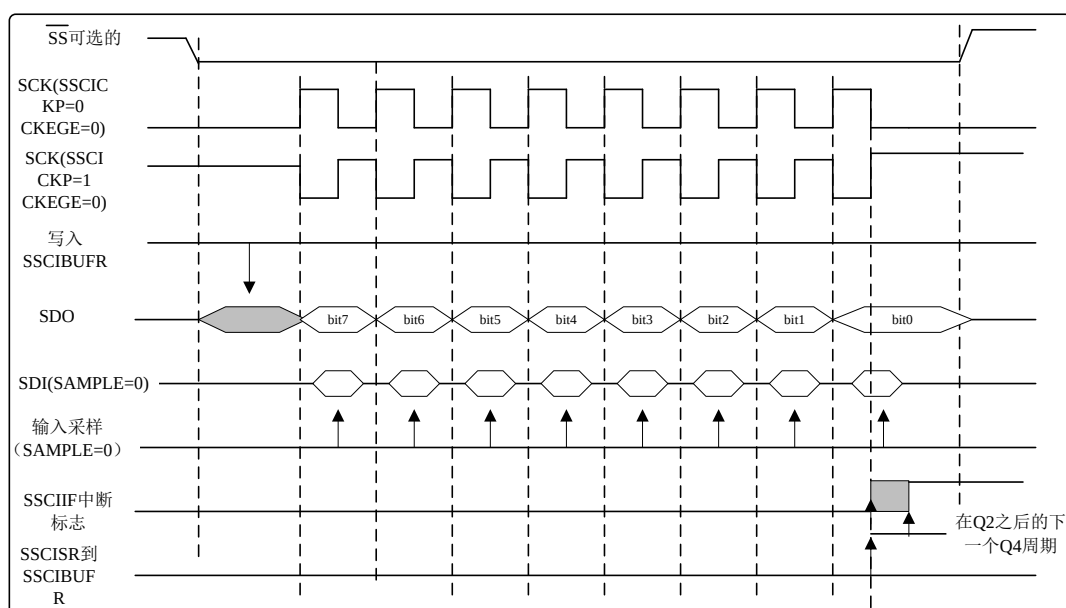
图 16.31 从动时序图
