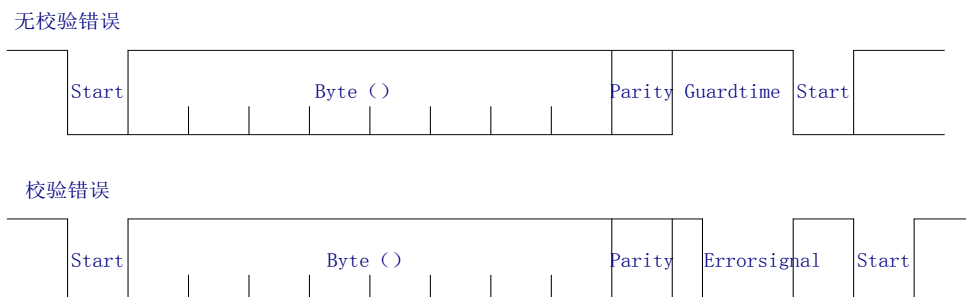
图 15.18 7816 接口时序
