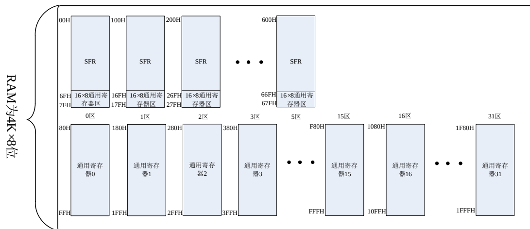
图 4.6 数据存储器地址映射图
