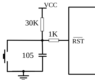
图 24.2 建议 \overline{\text{RST}} 复位电路
