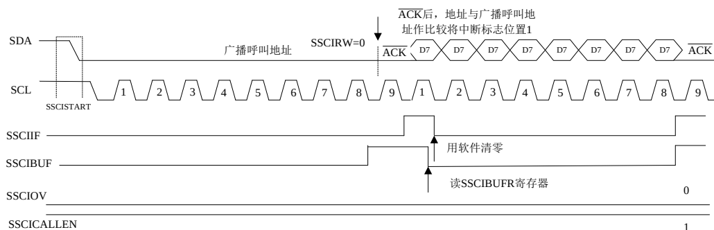
图 16.6 从动模式广播呼叫地址时序（7 或 10 位地址模式）
