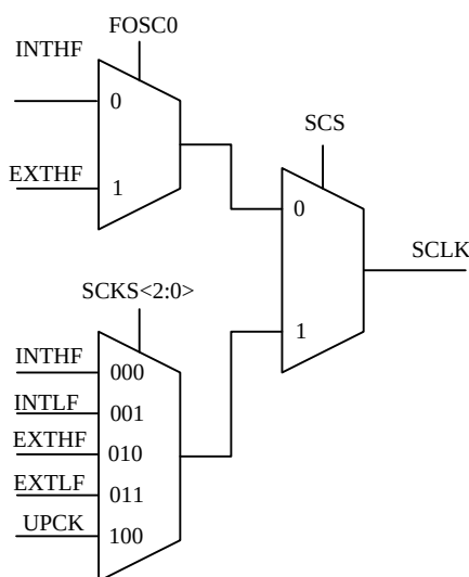
图 3.5 KF8F63XX 时钟模式选择
