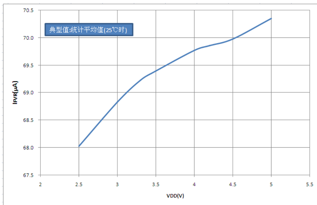
图 26.12: 欠压复位电流 I_{FVR} — V_{DD} 关系曲线图
