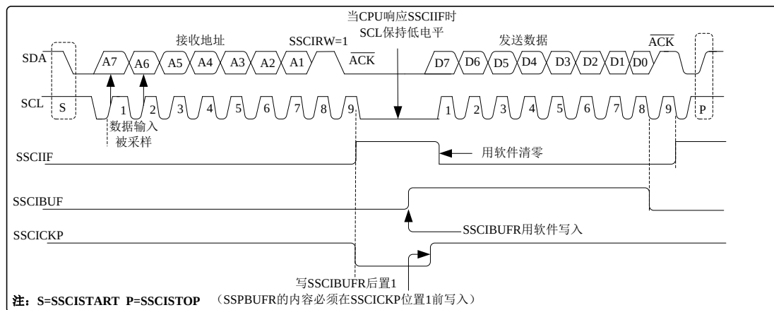
图 16.4 从动模式时序（发送，7 位地址）
