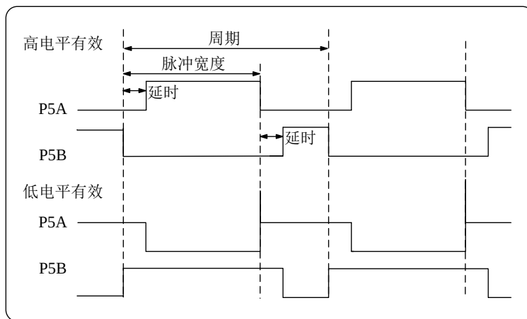
图 13.8 半桥输出模式输出信号示例
