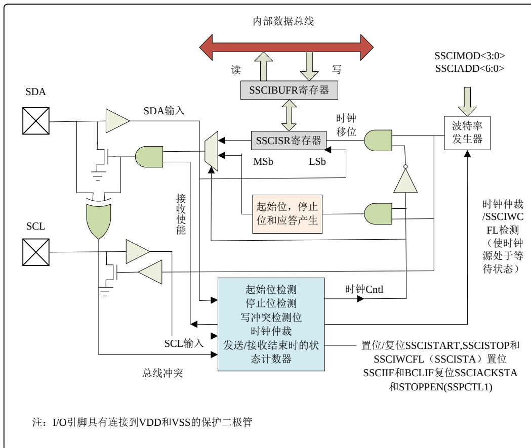
图 16.7为I2C主模式框图。
