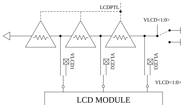
图 17.3 LCD 偏置电路原理框图
