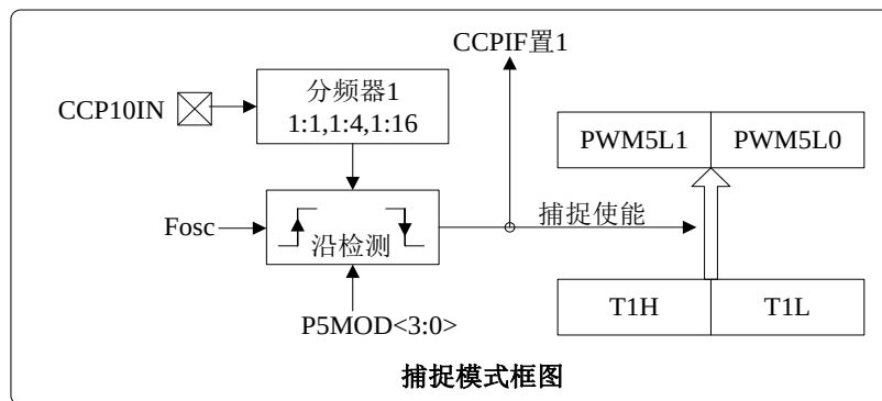
图 13.1 捕捉模式原理框图
