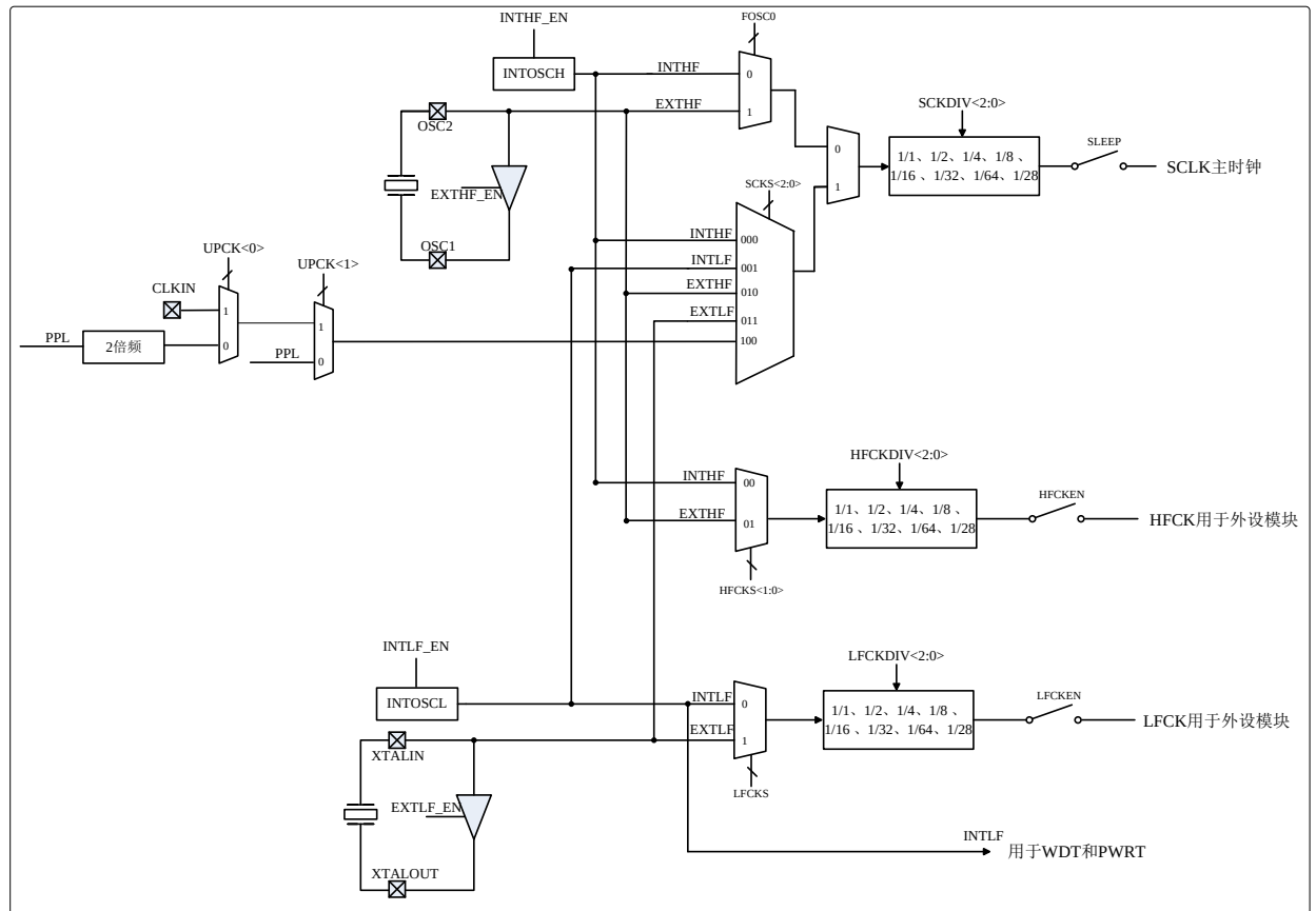
图 3.1 时钟模块原理框图
