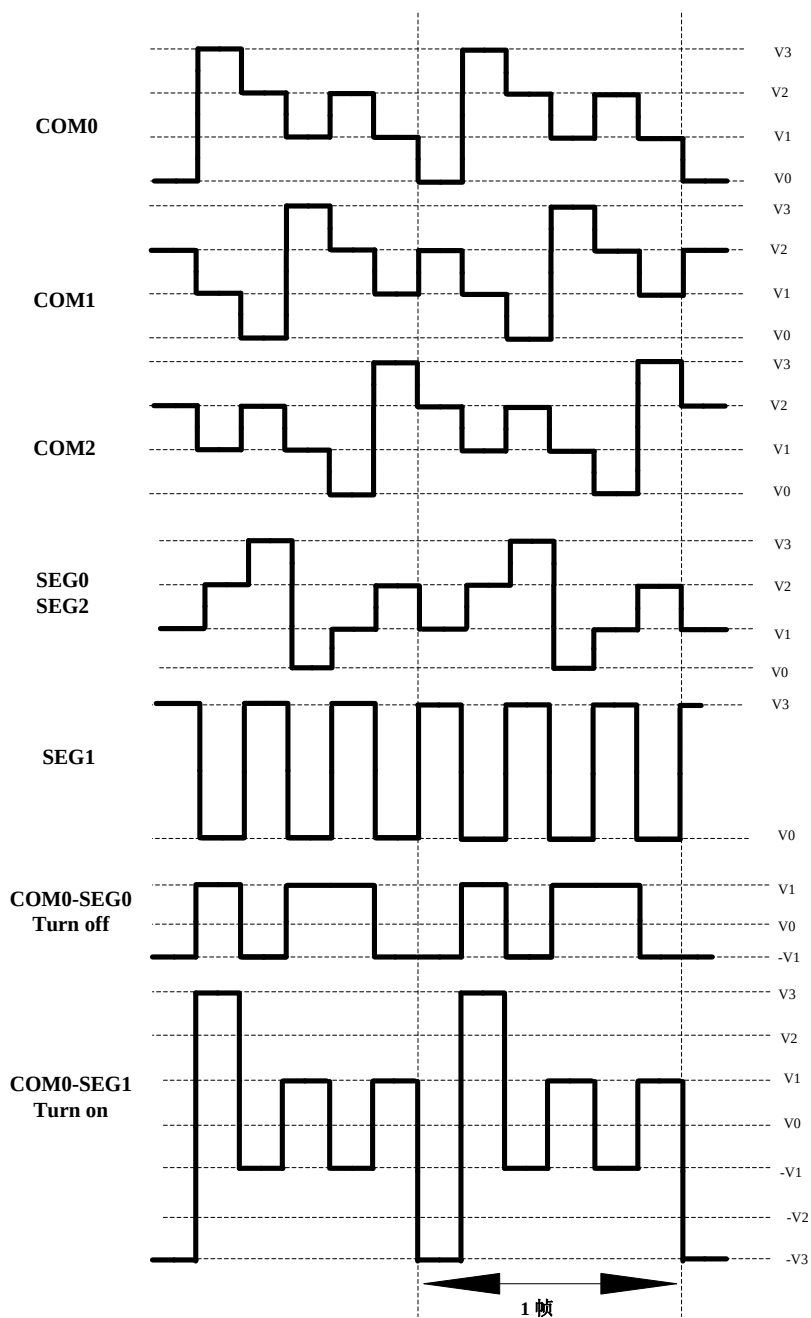
图 17.11 在 1/3 复用、1/3 偏置驱动时的 A 型波形
