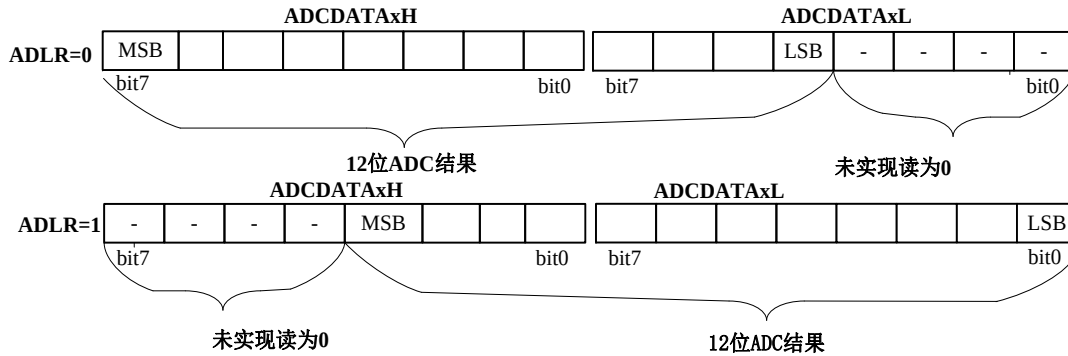
图 10.2 ADC 输出对齐方式
