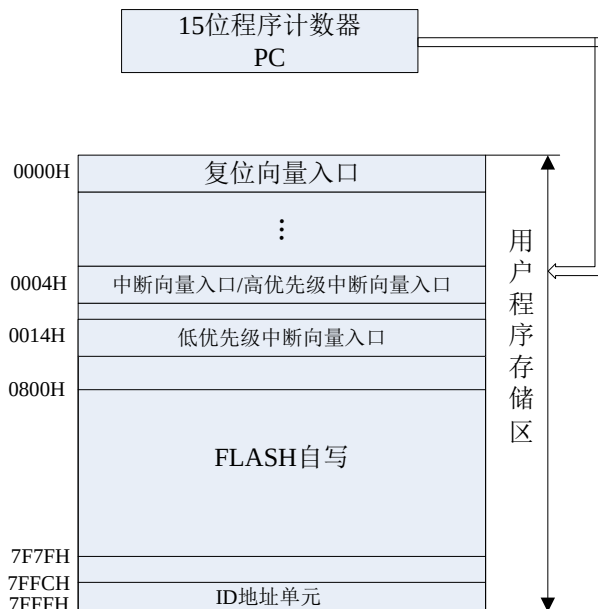
图 4.2 KF8F63XX 程序存储器映射
