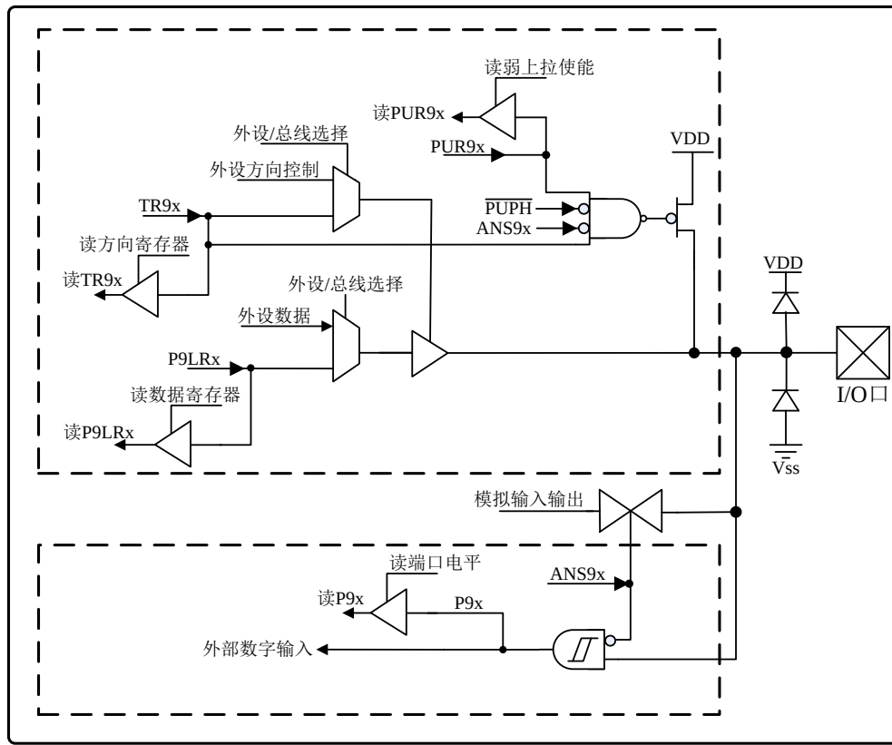
图 2.12 P9 口引脚原理功能框图
