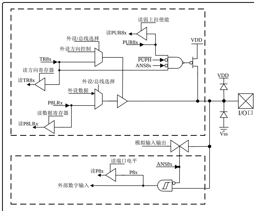
图 2.11 P8 口引脚原理功能框图
