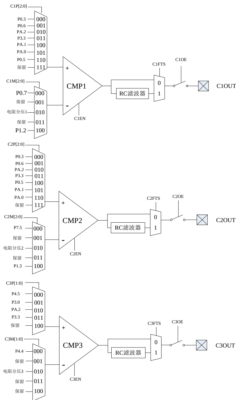
图 14.1 模拟比较器框图
