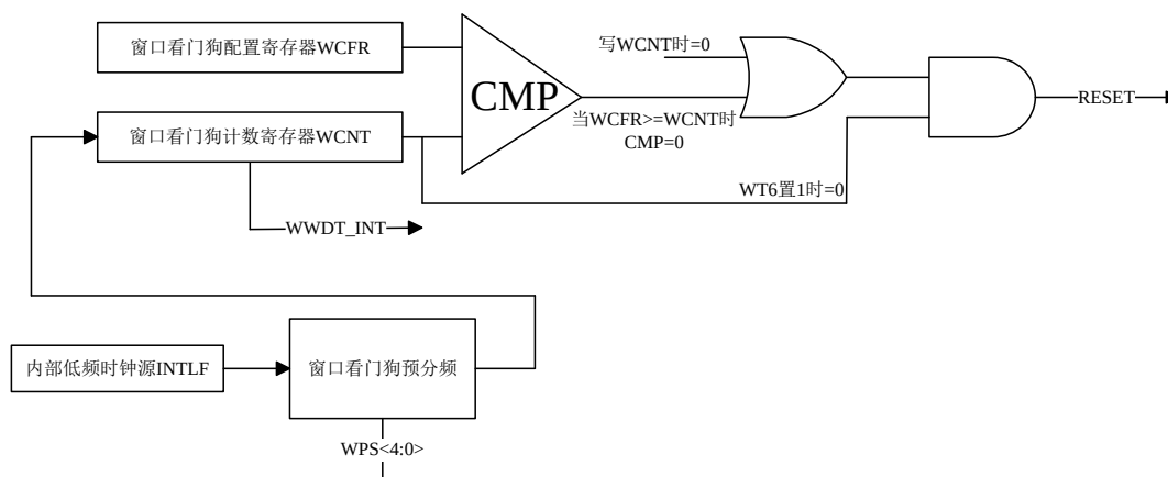
图 23.2 窗口看门狗原理框图
