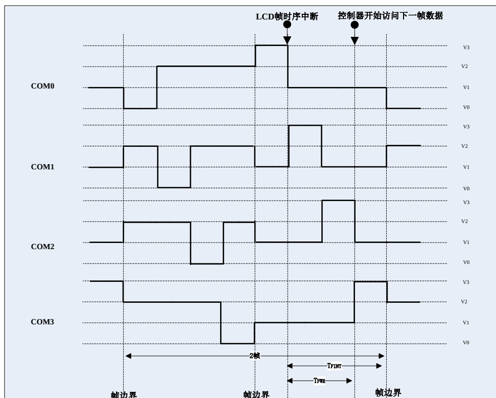
图 17.15 帧时序中断例图
