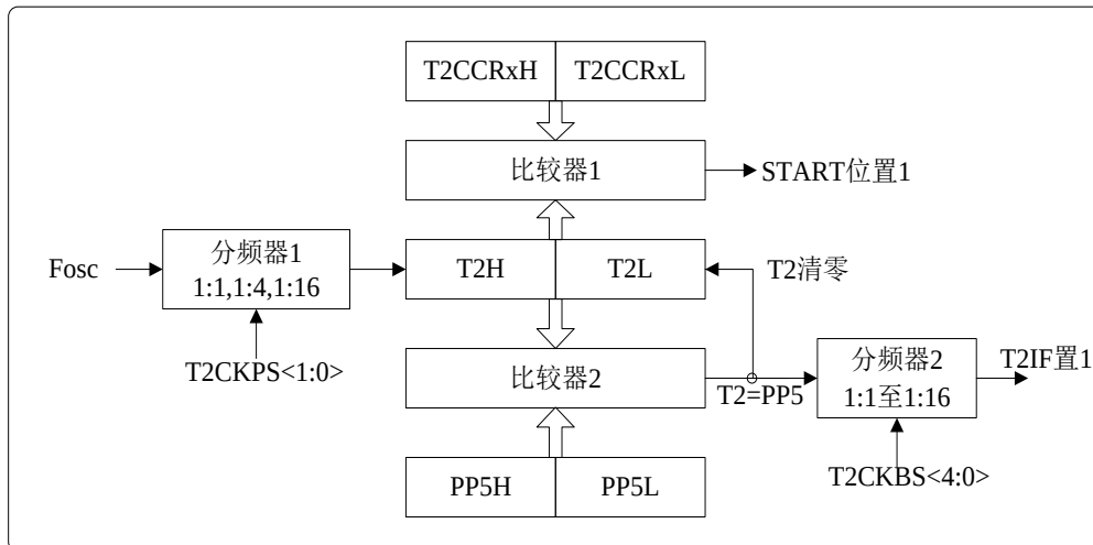
图 8.7 定时器 T10 原理框图
