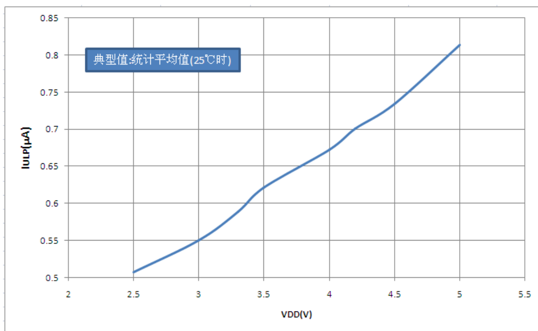
图 26.4: 不同 VDD 时典型 IULP — VDD 关系曲线图(超低功耗模式, 禁止所有外设)
