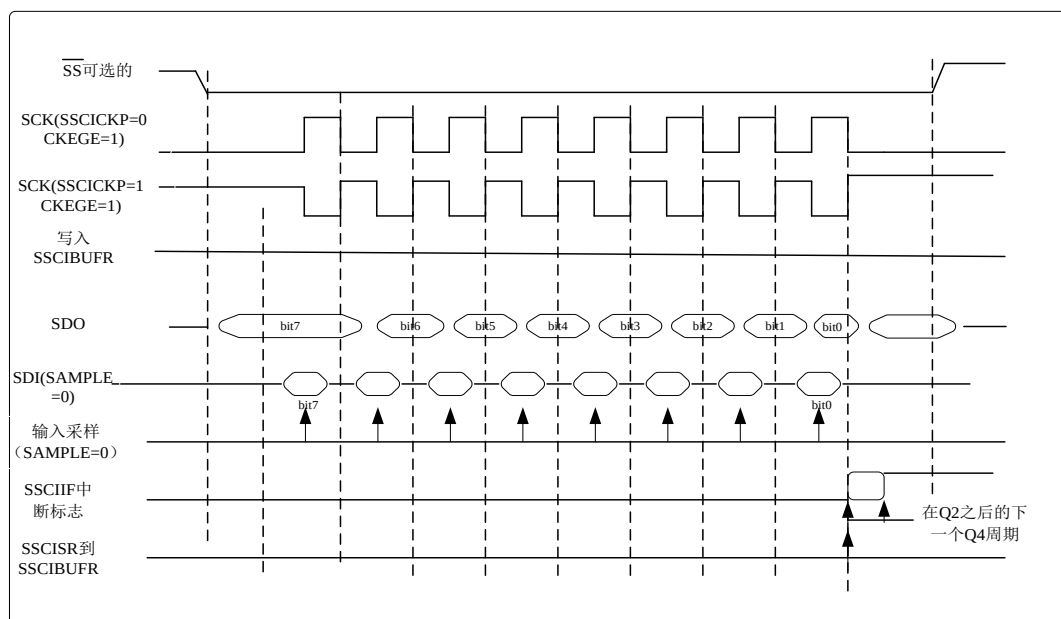
图 16.33 SPI 模式时序图（从动模式且 CKEGE=1）
