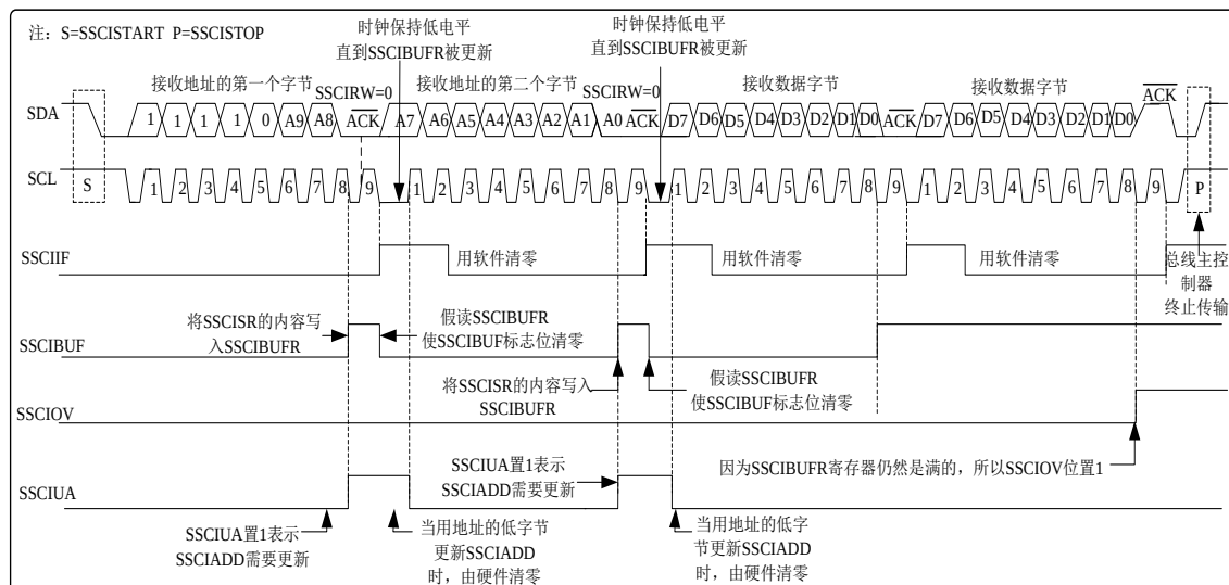
图 16.3 从动模式时序（接收，10 位地址）
