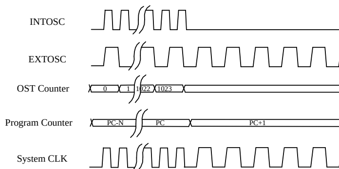
图 3.7 双速启动时序
