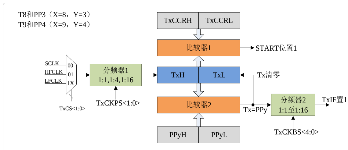
图 8.6 定时器 T8 原理框图
