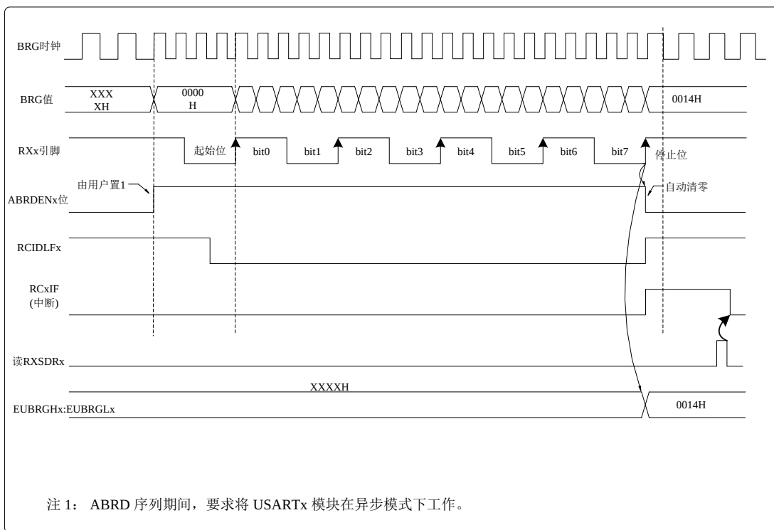
图 15.3 自动波特率检测
