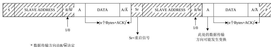
图 16.11 I2C 协议复合数据帧格式
