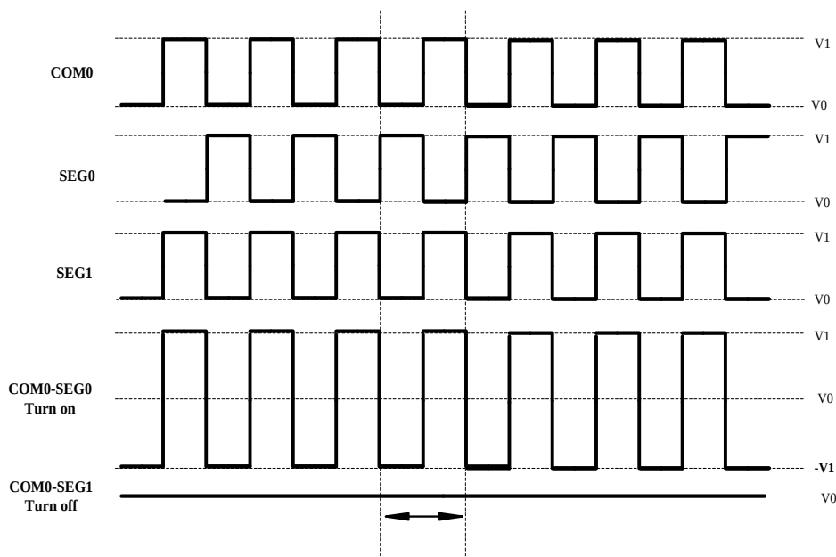
图 17.4 在静态驱动时 A/B 型波形
