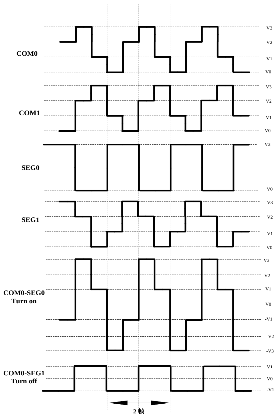
图 17.8 在 1/2 复用、1/3 偏置驱动时的 B 型波形
