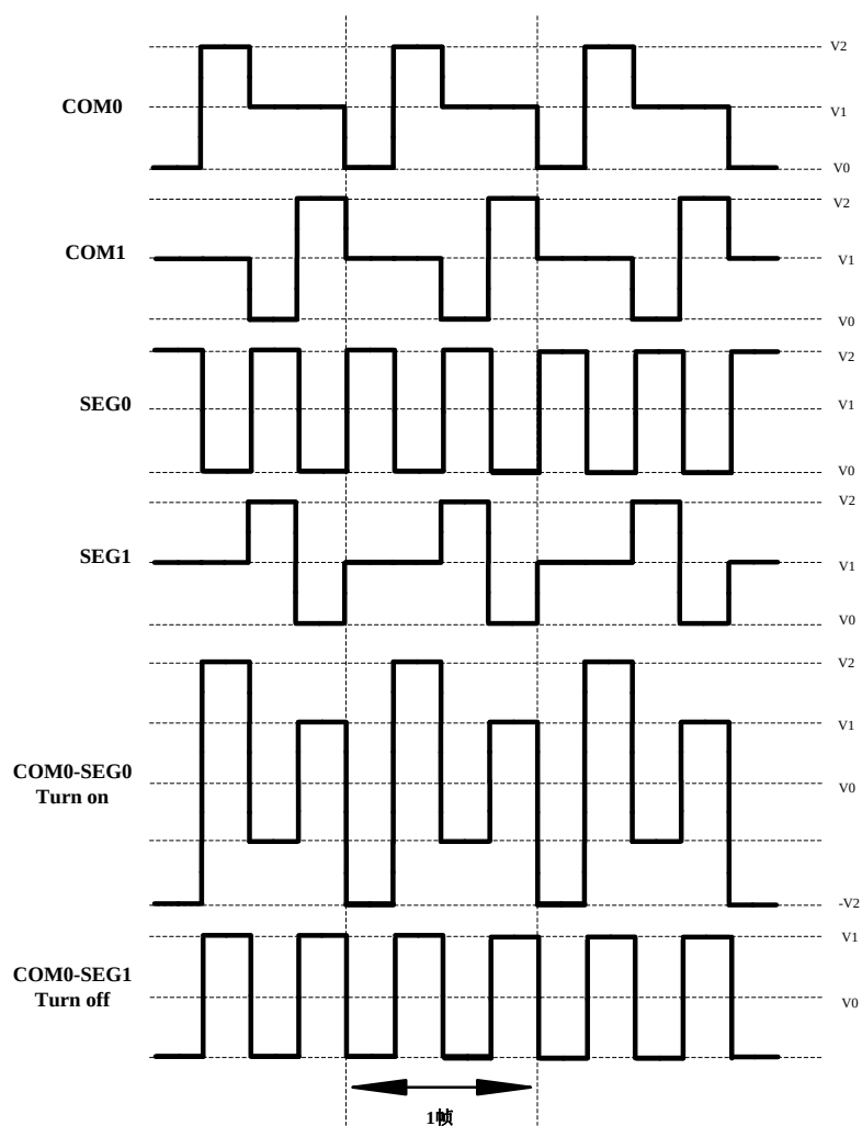
图 17.5 在 1/2 复用、1/2 偏置驱动时的 A 型波形
