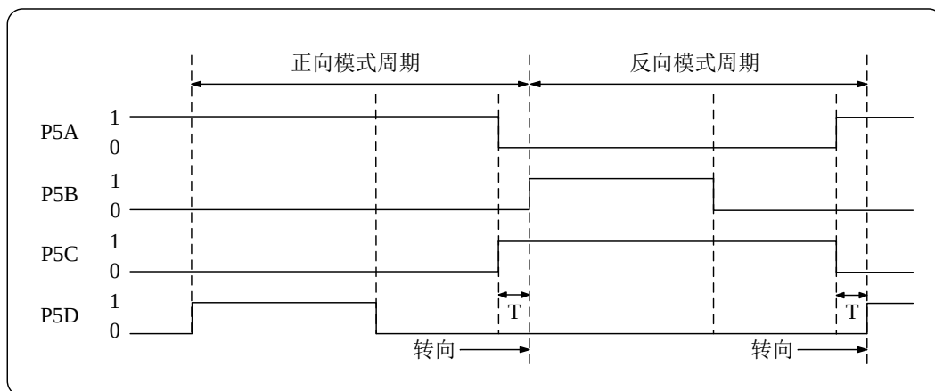
图 13.14 全桥正向、反向输出模式转换示例(高电平有效)
