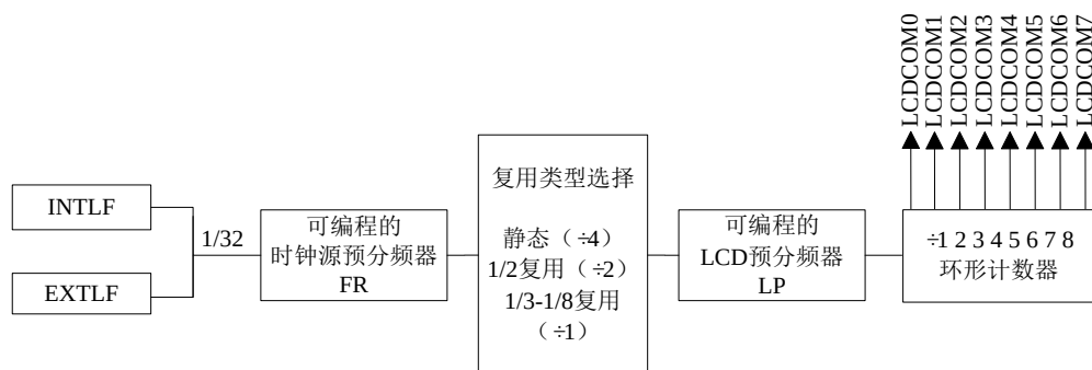
图 17.2 LCD 预分频器图
