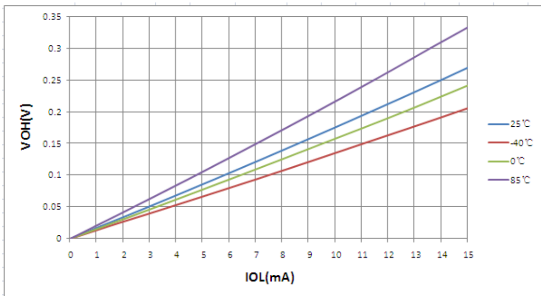
图 26.16:不同温度时 V_{OH} — I_{OL} 关系曲线图 ( V_{DD} = 3.0V )
