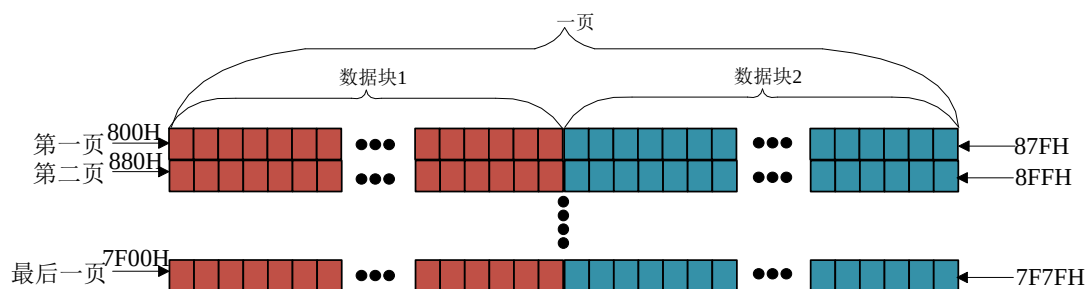
图 4.7 Flash 自写区域地址映射图
