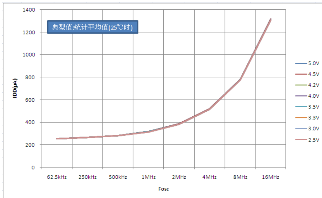
图 26.1: 不同 VDD 时典型 I DD — F osc 关系曲线图(HFINTOSC 模式)
