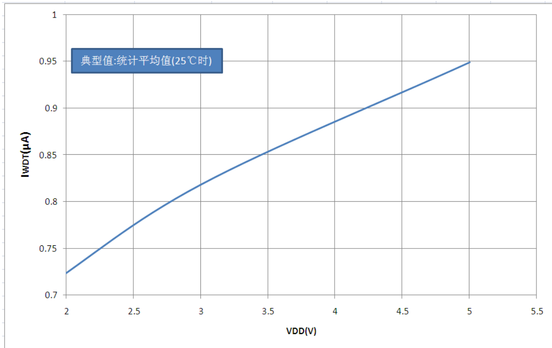
图 26.7:看门狗电流 I_{WDT} — V_{DD} 关系曲线图
