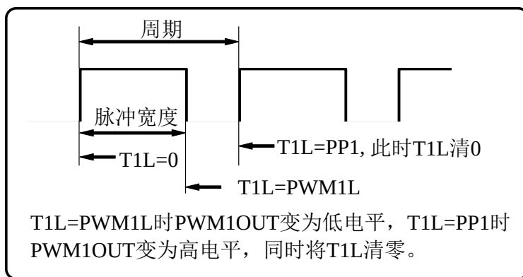
图 11-1 PWM1OUT 输出波形图
