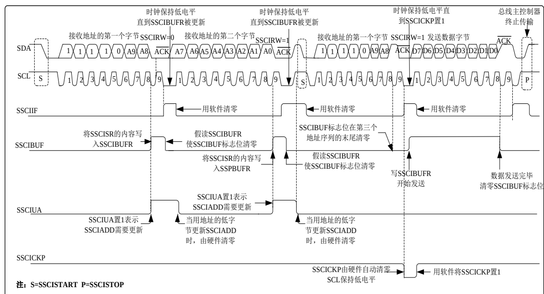
图 16.5 从动模式时序（发送，10 位地址）
