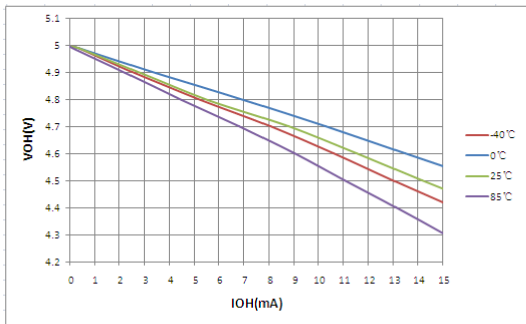
图 26.13:不同温度时 V_{OH} — I_{OH} 关系曲线图 ( V_{DD} = 5.0V )
