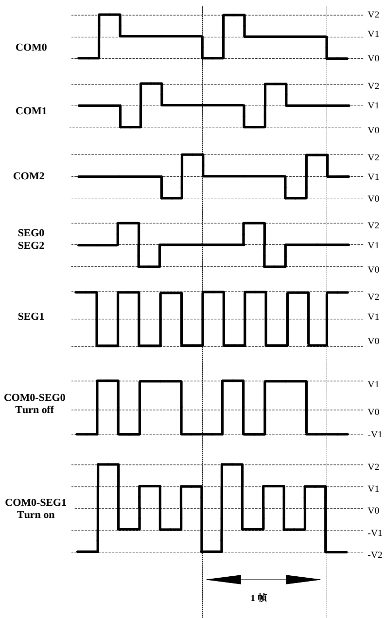
图 17.9 在 1/3 复用，1/2 偏置驱动时的 A 型波形
