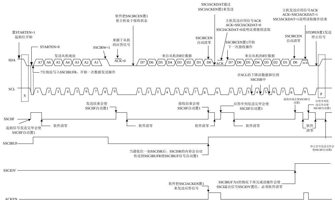
图 16.16为典型读数据帧格式在单片机硬件I2C上的实现接收过程时序图。
