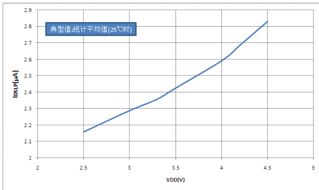
图 26.3: 不同 VDD 时典型 IDSLP — VDD 关系曲线图(深度休眠模式, 禁止所有外设)
