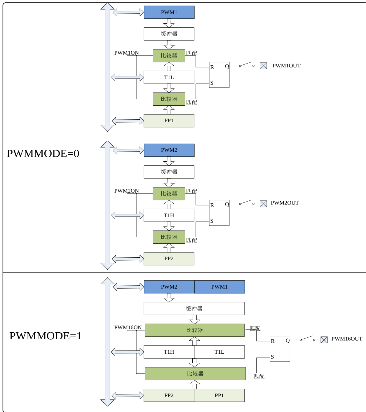
图 11.1 PWM 逻辑框图
