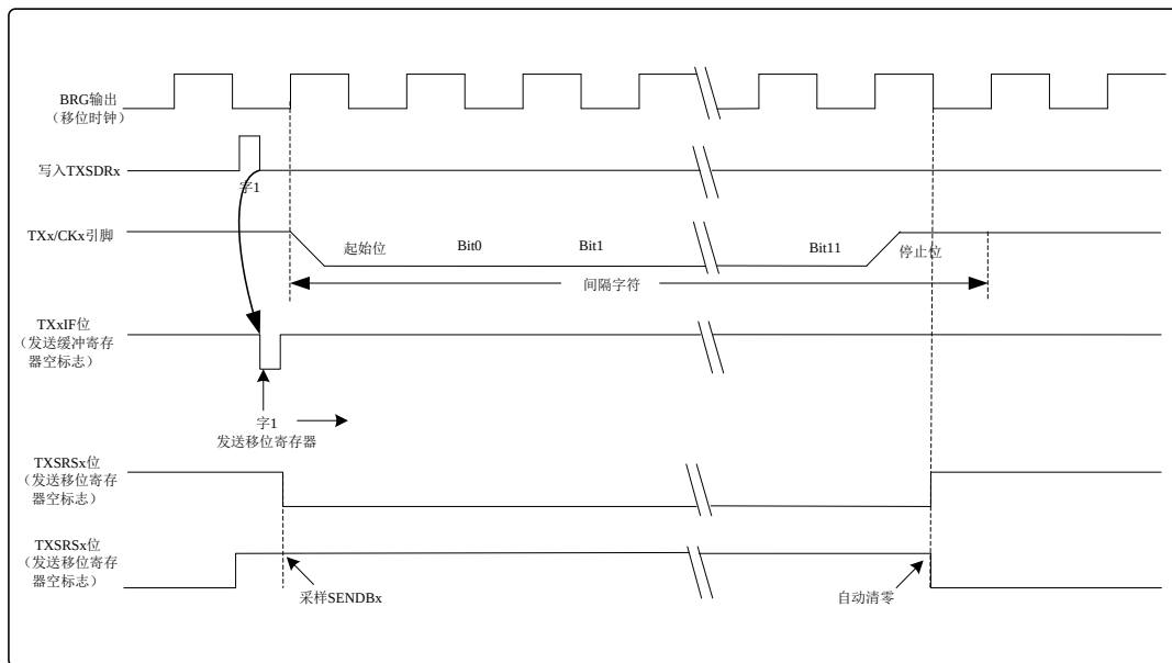
图 15.6 发送间隔字符时序
