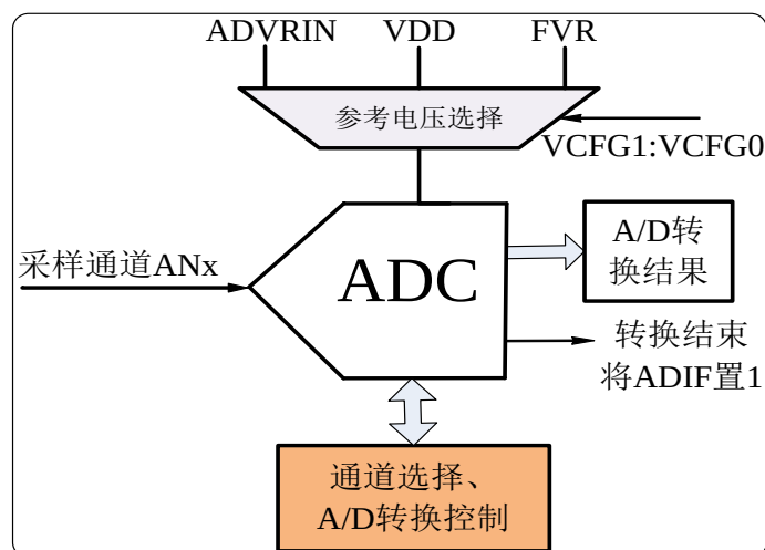
图 10.1 AD 模块结构框图
