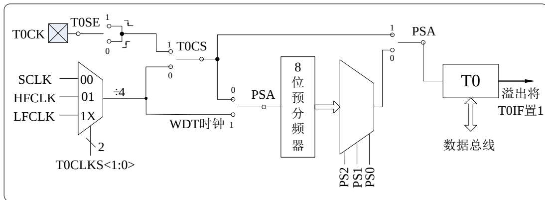
图 8.1 原理框图
