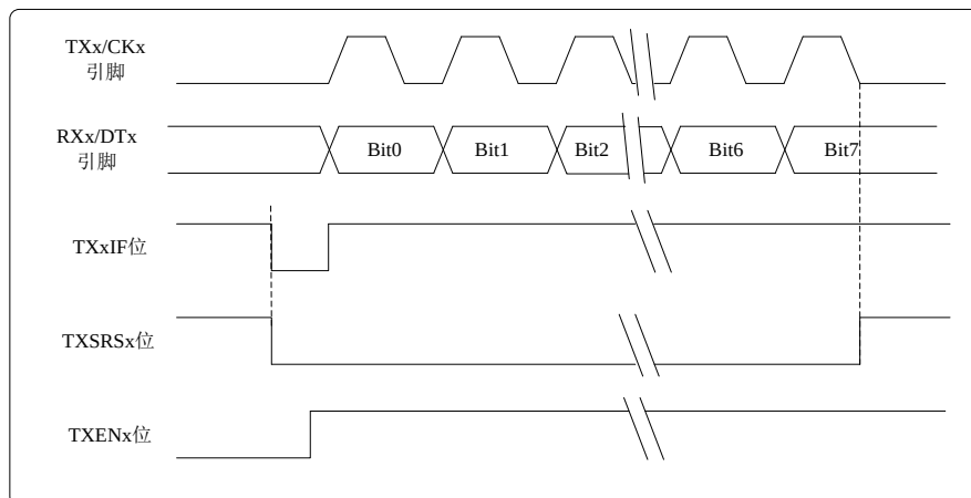
图 15.14 半双工同步发送（通过 TXENx）
