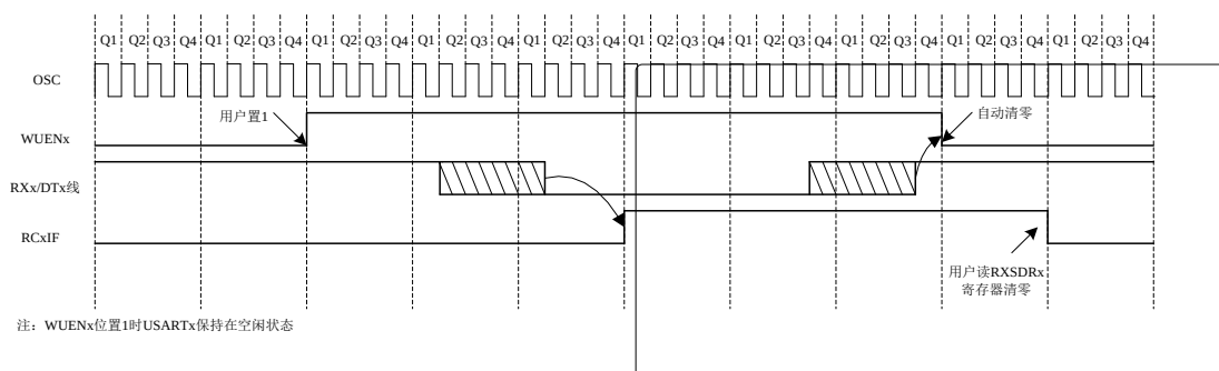
图 15.4 正常工作下的自动唤醒时序
