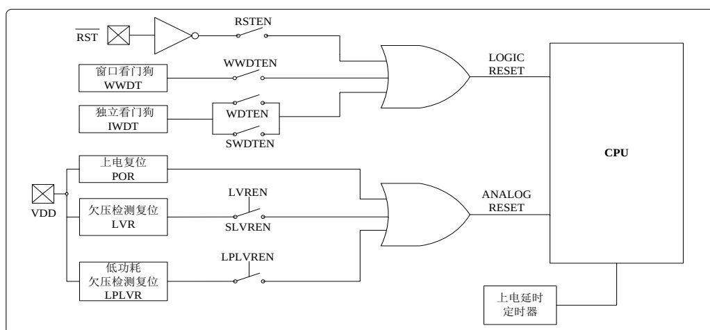
图 24.1 片内复位电路简化框图
