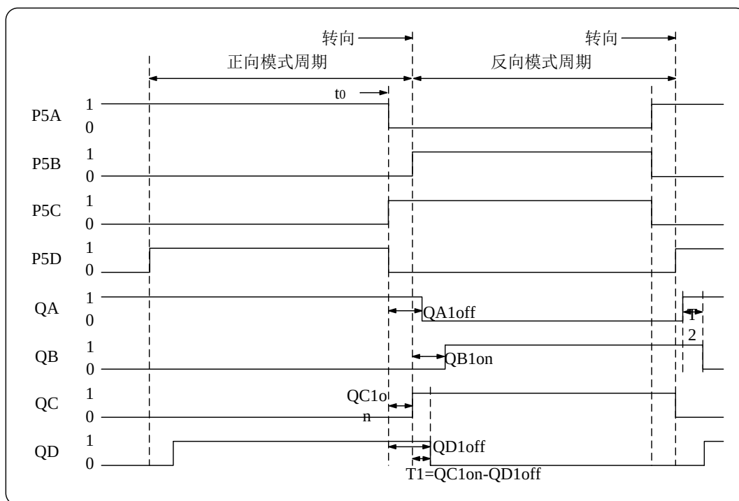
图 13.15 接近满占空比时换向时信号示例
