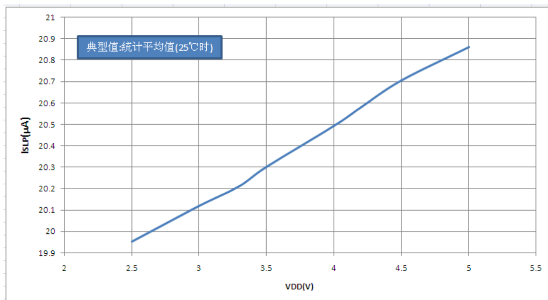
图 26.2: 不同 VDD 时典型 I SLP — VDD 关系曲线图(普通休眠模式, 禁止所有外设)
