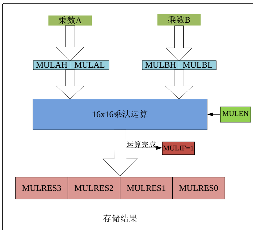
图 18.1 16×16 硬件乘法器原理框图
