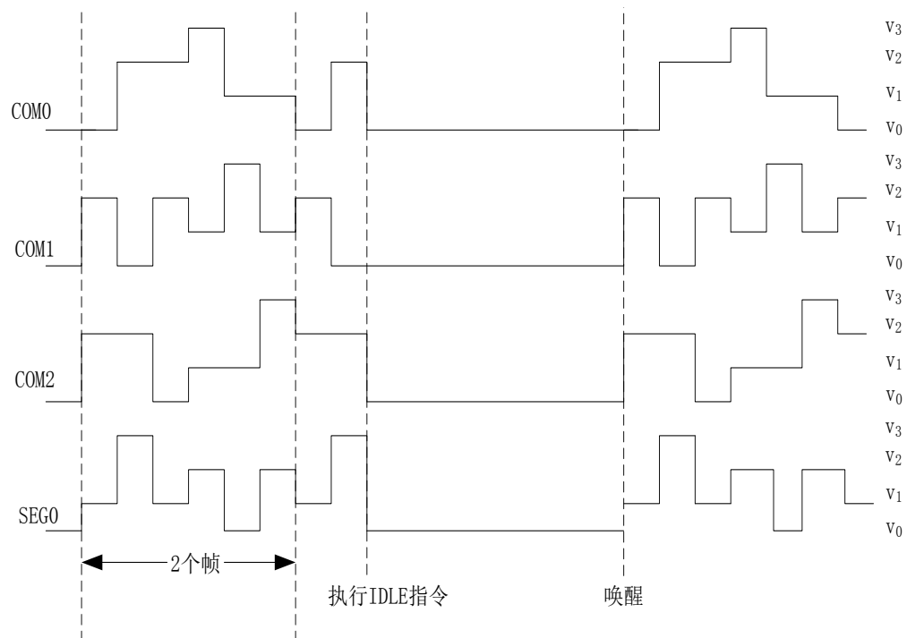
图 17.16 当 \overline{\text{SLPEN}} = 1 是进入/退出休眠模式
