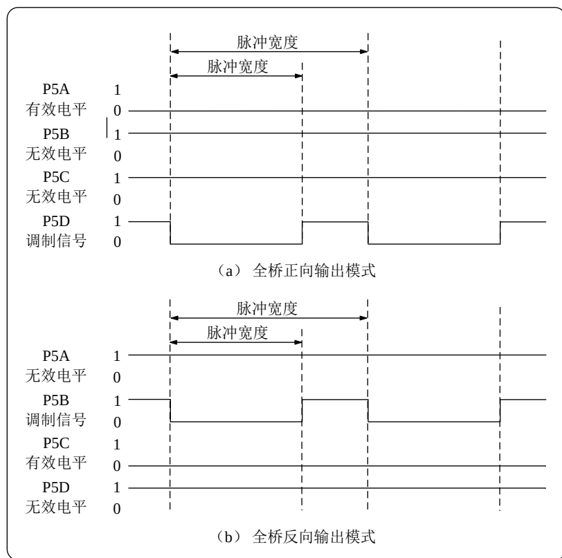
图 13.11 全桥输出模式引脚信号示例(高电平有效)
