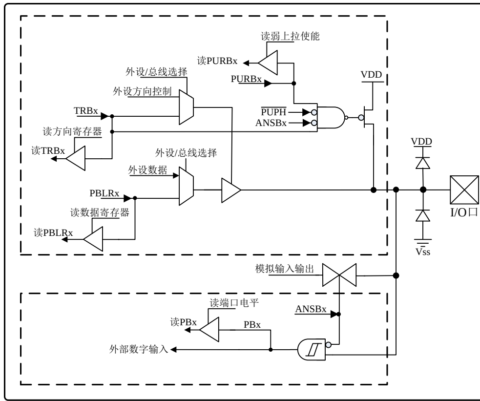
图 2.14 PB 口引脚原理功能框图
