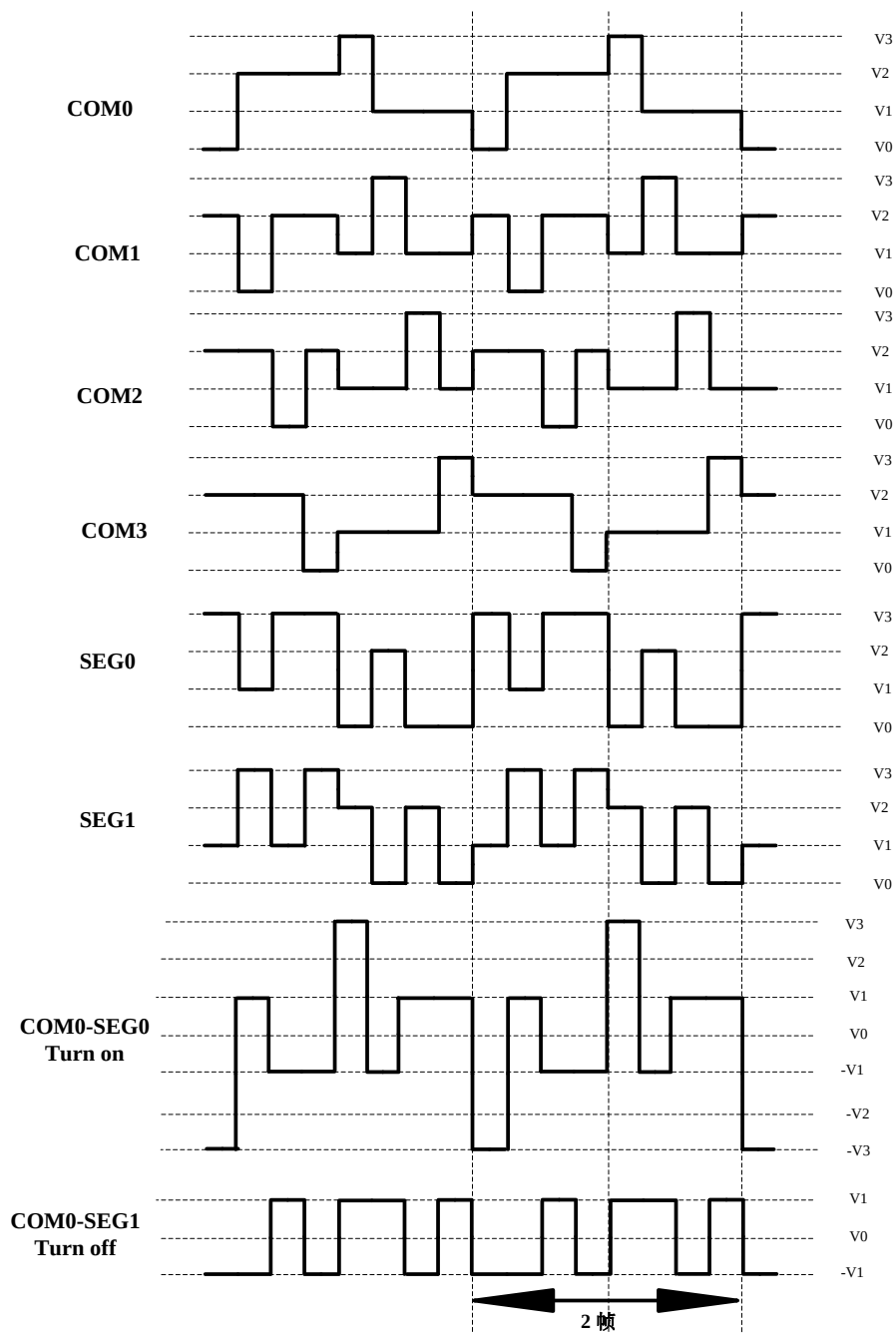
图 17.14 在 1/4 复用、1/3 偏置驱动时的 B 型波形
