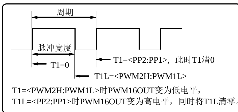
图 11-2 PWM1OUT 输出波形图
