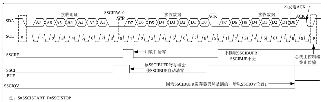
图 16.2 从动模式时序（接收，7 位地址）
