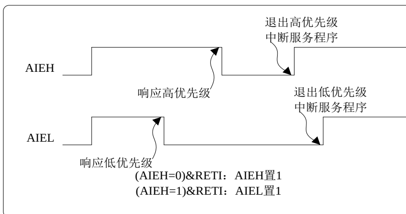
图 6.1 中断优先级工作原理图
