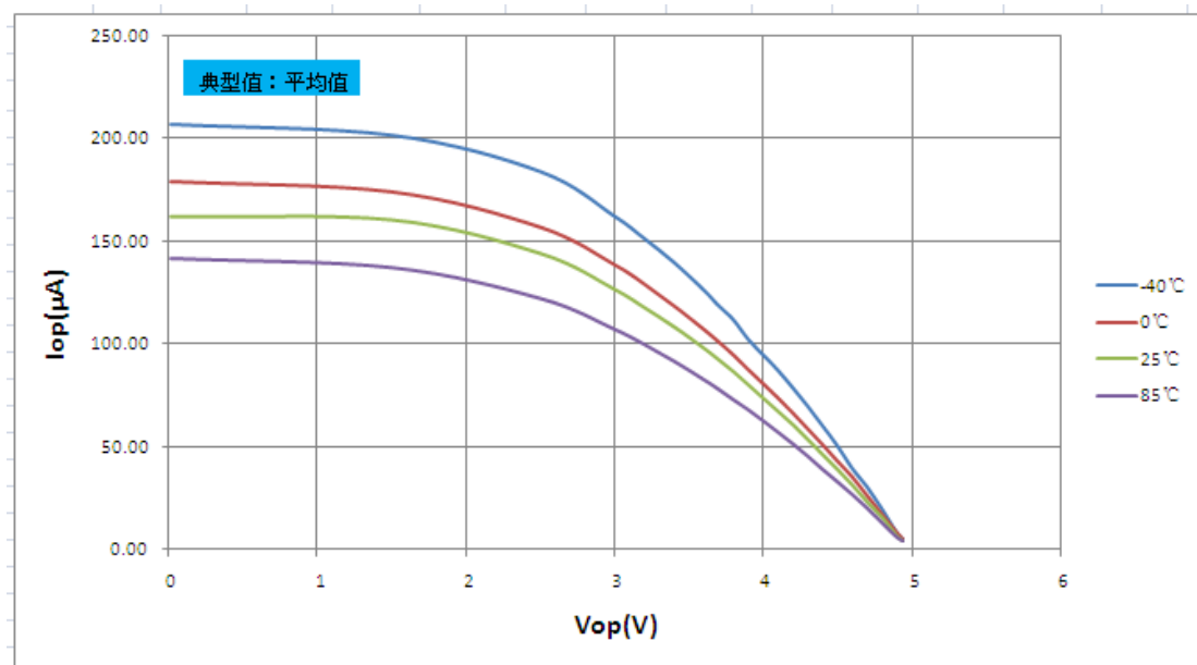
图 26.17:上拉功能打开时端口电压 V_{OP} — 电流 I_{OP} 关系曲线图 ( V_{DD} = 5.0V )
