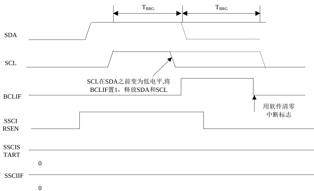
图 16.25 重复启动条件期间的总线冲突（情形 2）
