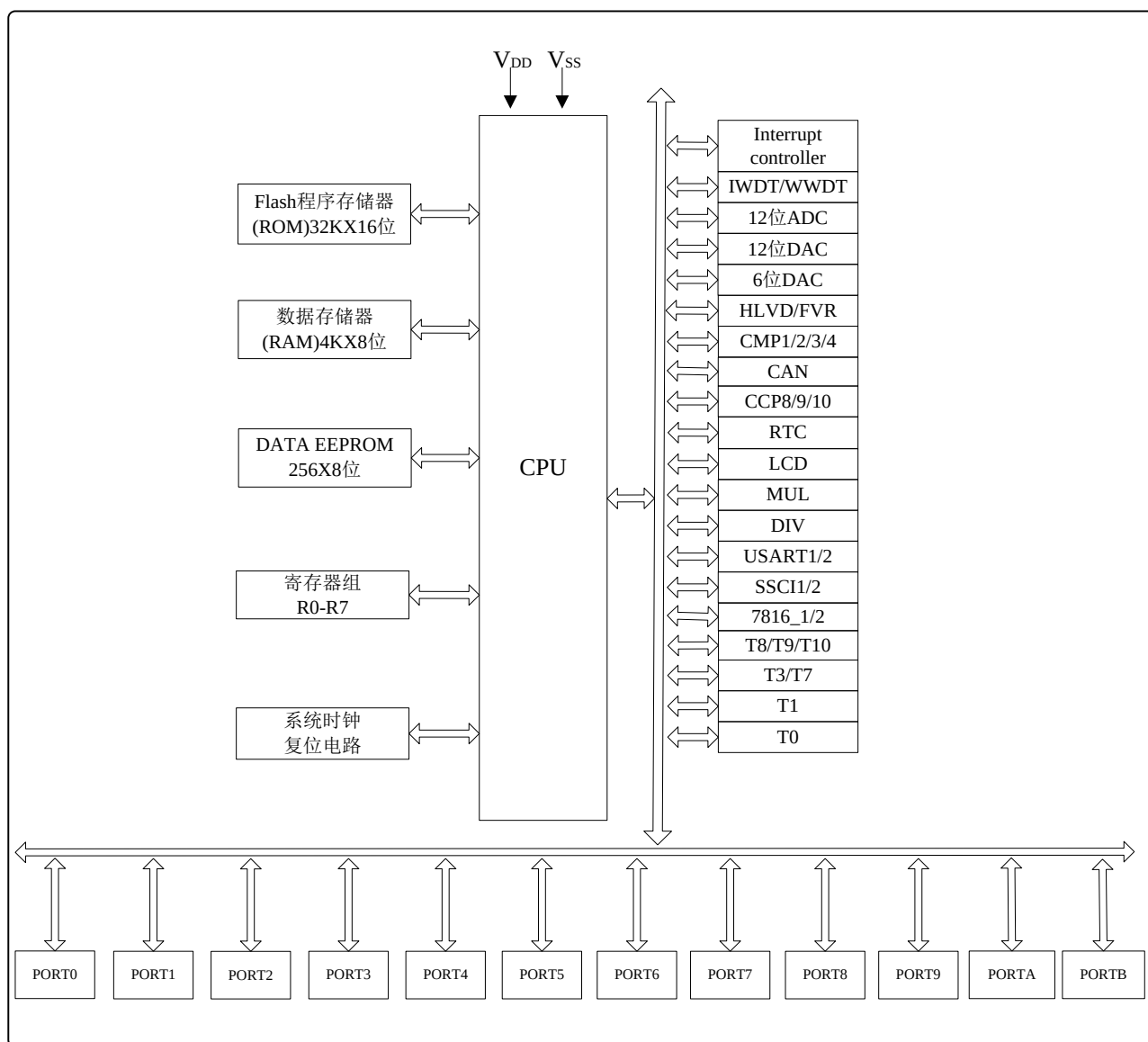
图 1.1KF8F63XX 单片机系统框图
