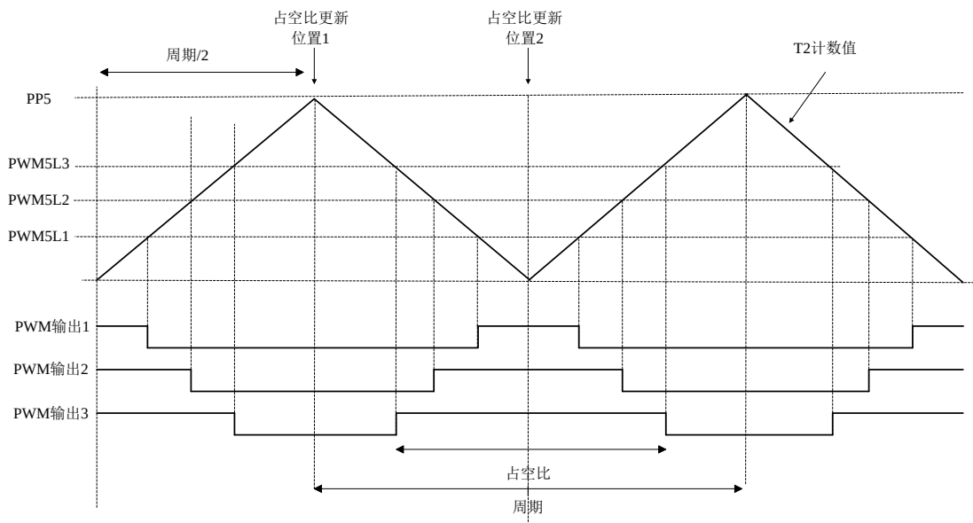
图 13.5 中心对齐 PWM
