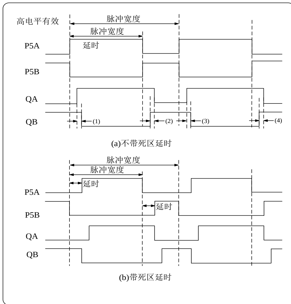
图 13.10 带死区控制和不带死区控制时的信号示例
