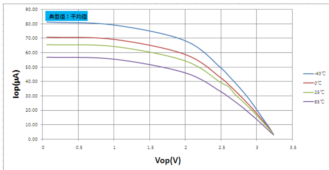
图 26.18:上拉功能打开时端口电压 V_{OP} — 电流 I_{OP} 关系曲线图 ( V_{DD} = 3.3V )
