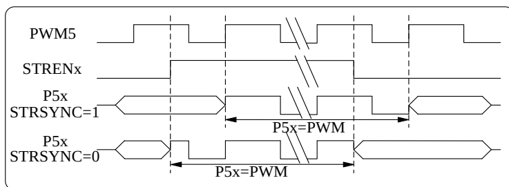
图 13.7 单输出模式 PWM 输出引脚切换
