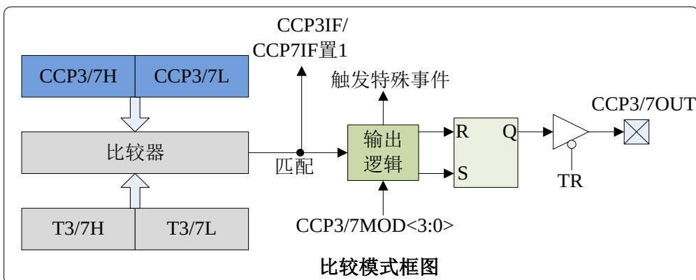
图 8.5 比较模式原理框图
