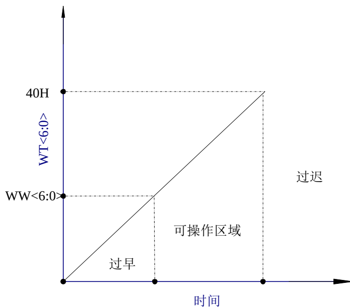
图 23.3 窗口看门狗原理图
