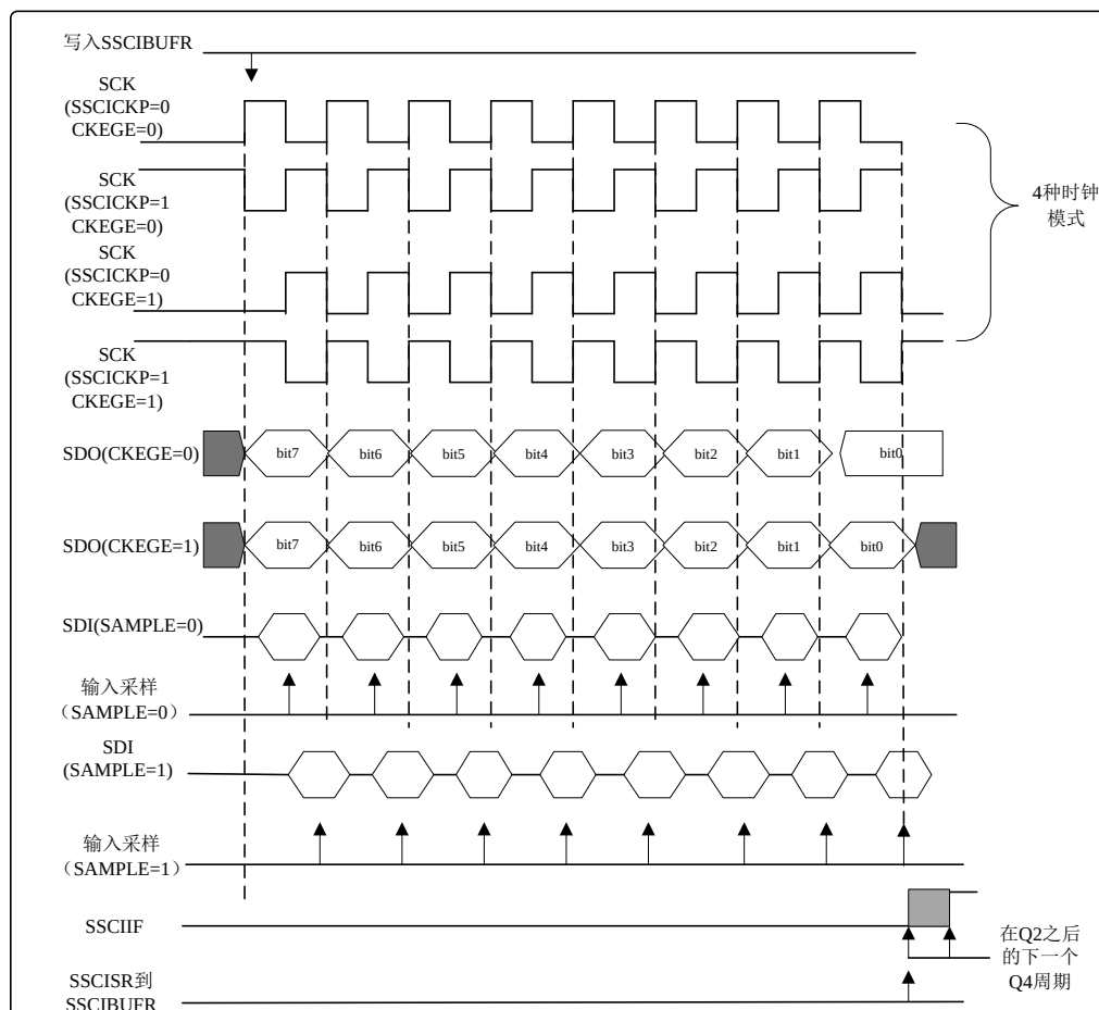
图 16.30 SPI 主控模式时序图
