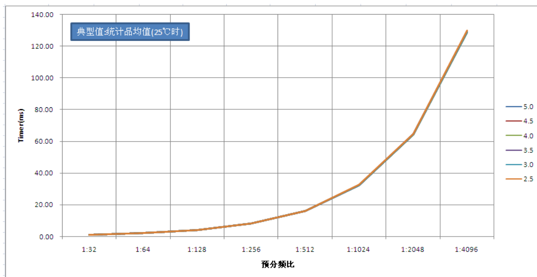
图 26.6: 不同 VDD 时看门狗预分频比 PS<2:0> 一周关系曲线图
