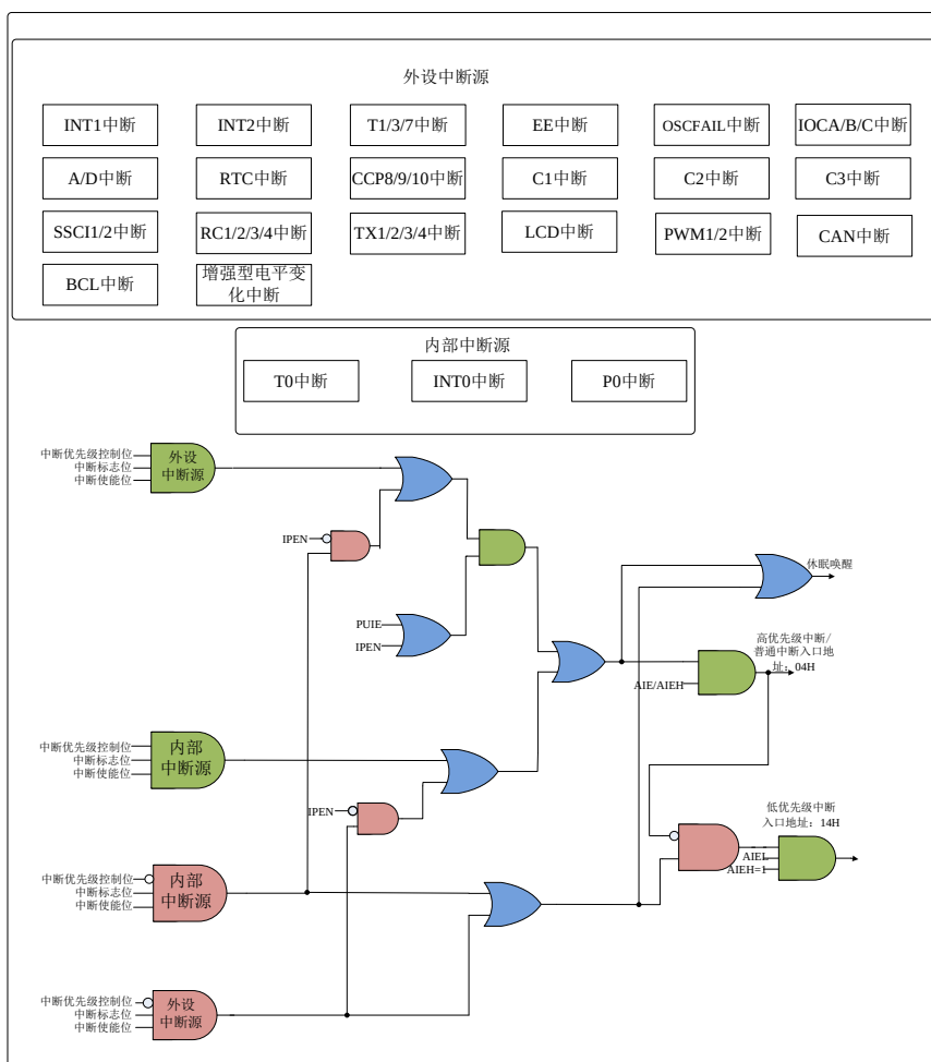
图 6.2 中断逻辑
