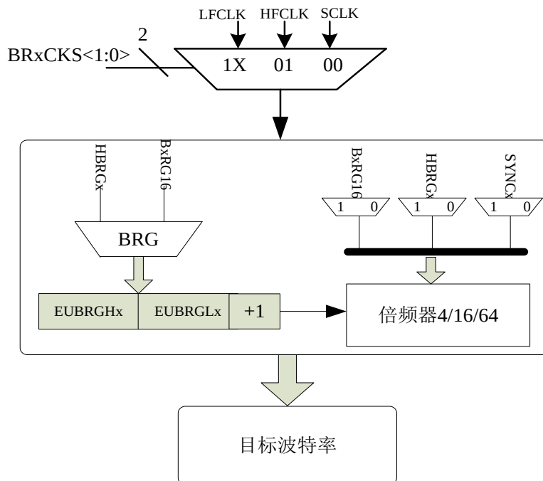
图 15.2 USARTx 目标波特率产生原理框图
