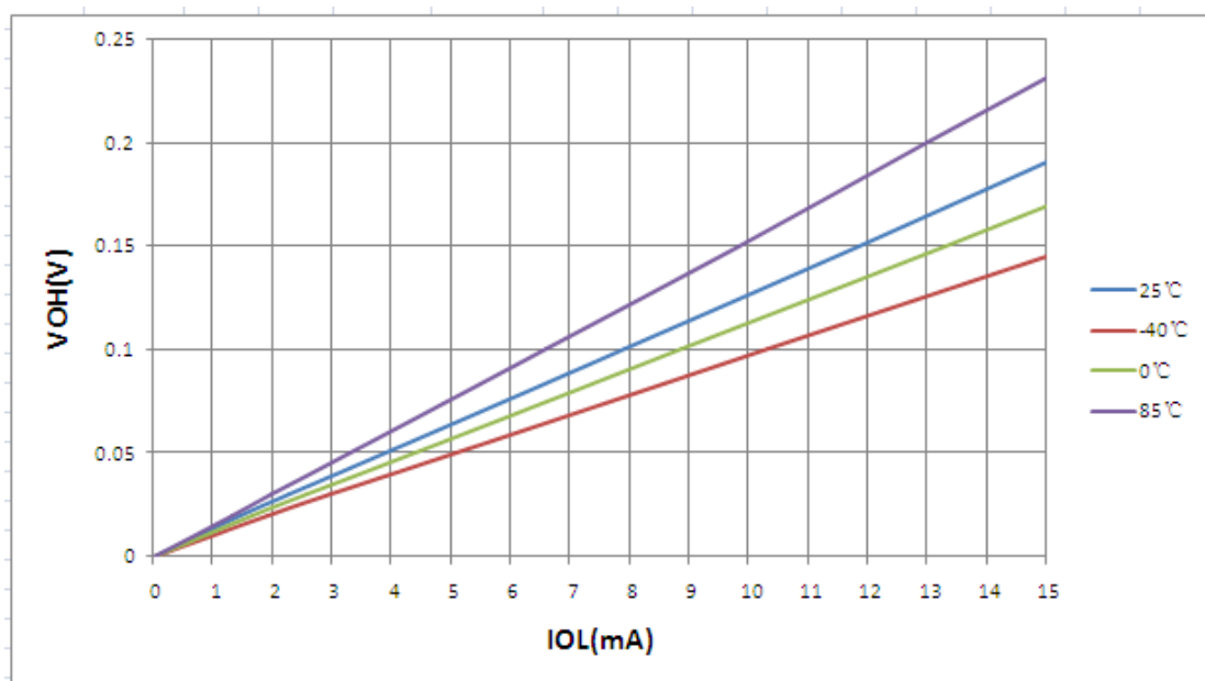
图 26.15:不同温度时 V_{OH} — I_{OL} 关系曲线图 ( V_{DD} = 5.0V )
