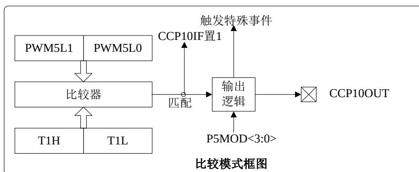
图 13.2 比较模式原理框图
