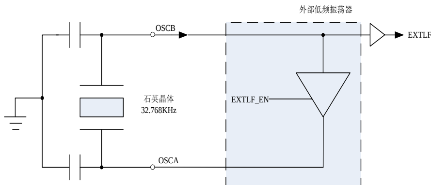
图 1.4 EXTLF 原理图
