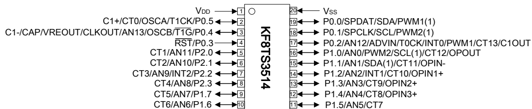
SOIC-20 引脚示意图:
