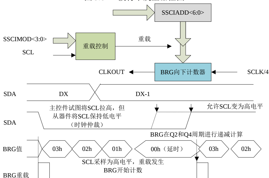
图 9.9 带有时钟仲裁的波特率发生器时序
