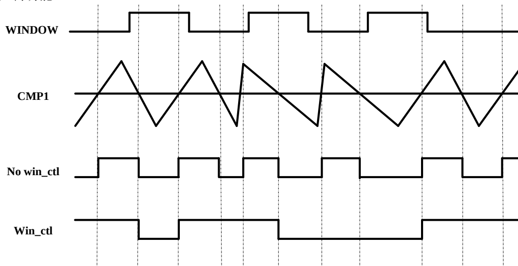
图 11.2 模拟比较器范围控制
