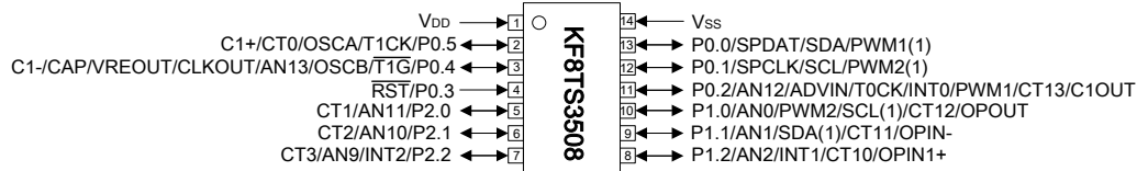
SOIC-14 引脚示意图:
