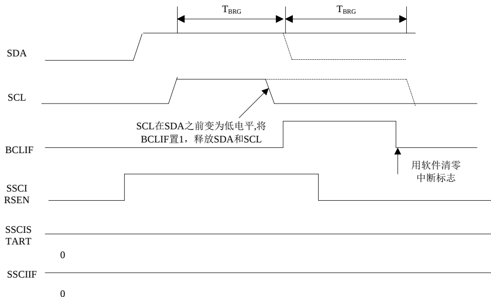
图 9.25 重复启动条件期间的总线冲突（情形 2）
