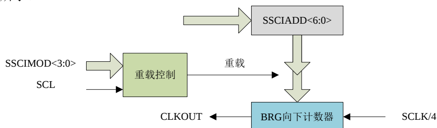
图 9.8 波特率发生器框图
