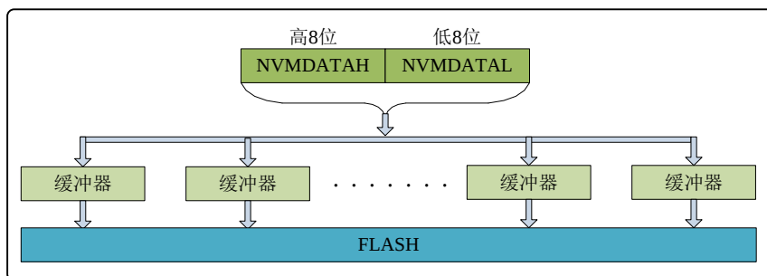
图 3.7 写操作
