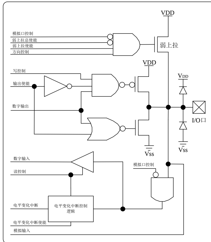
图 2.3 P0.0~P0.2、P0.4~P0.5 口引脚原理框图
