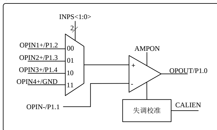
图 12.1 运放内部框图
