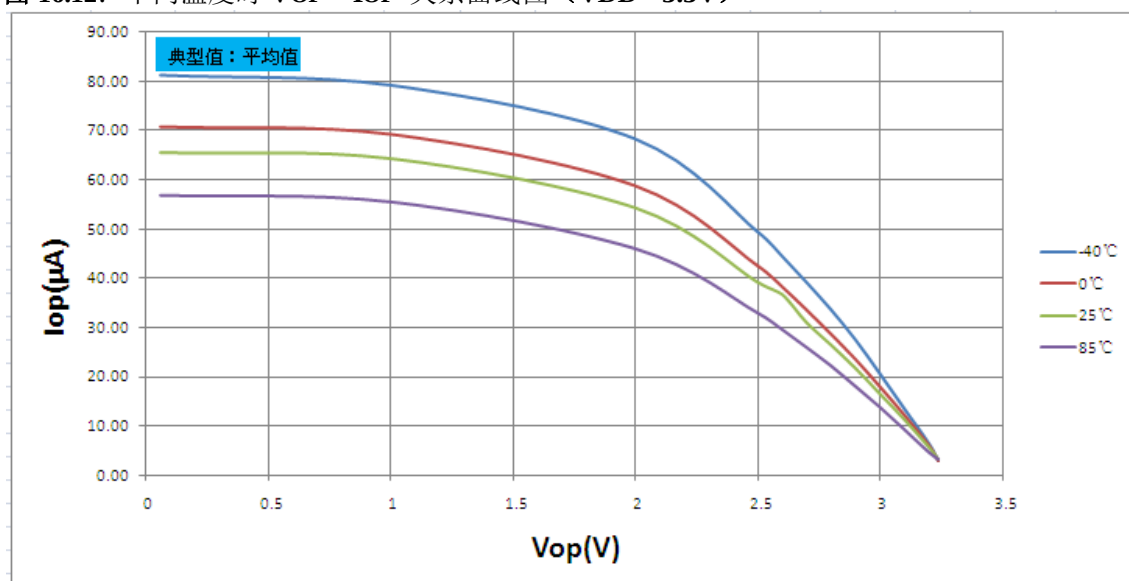
图 16.12: 不同温度时 VOP—IOP 关系曲线图 (VDD =3.3V)
