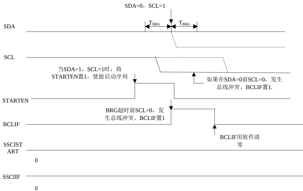
图9.22 启动条件期间的总线冲突（SCL=0）
