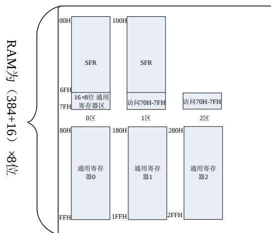
图 3.4 数据存储器地址映射图
