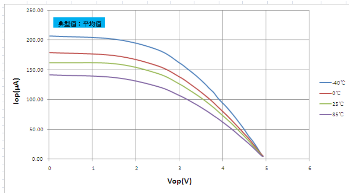
图16.11: 不同温度时VOP—IOP 关系曲线图 (VDD =5.0V)
