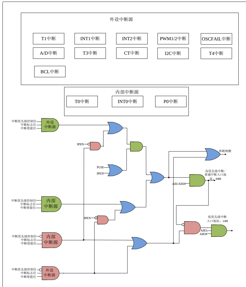
图 5.2 中断逻辑
