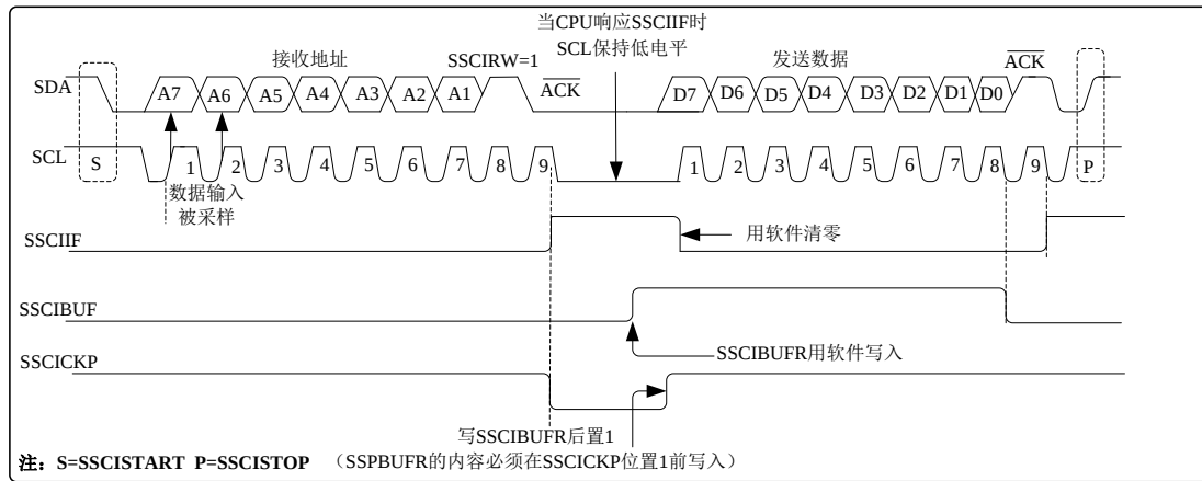
图 9.4 从动模式时序（发送，7 位地址）
