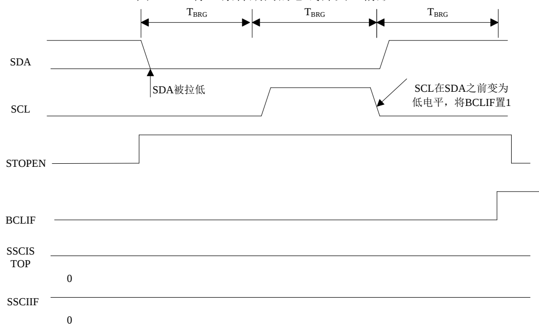
图9.25 停止条件期间的总线冲突(情形2)
