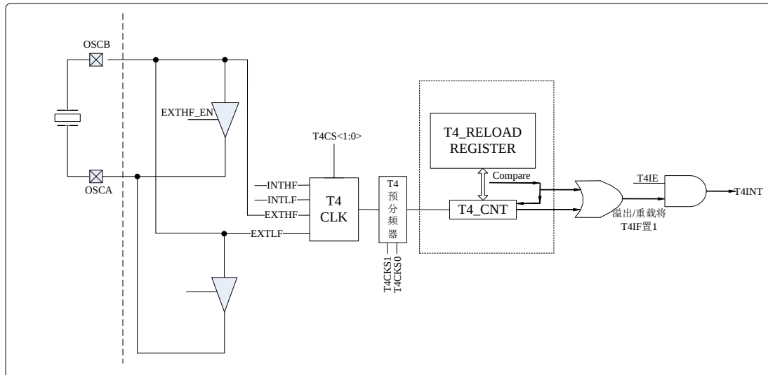
图 6.3 T4 原理框图
