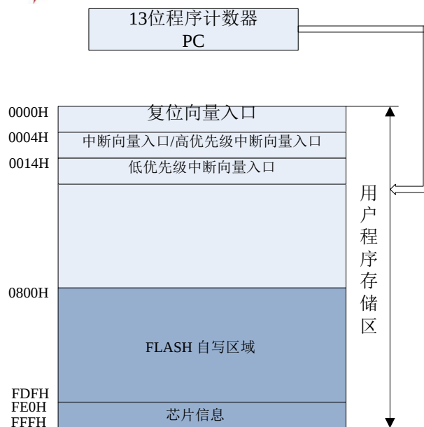
图 3.3 KF8TS3508/3510/3514 程序存储器映射
