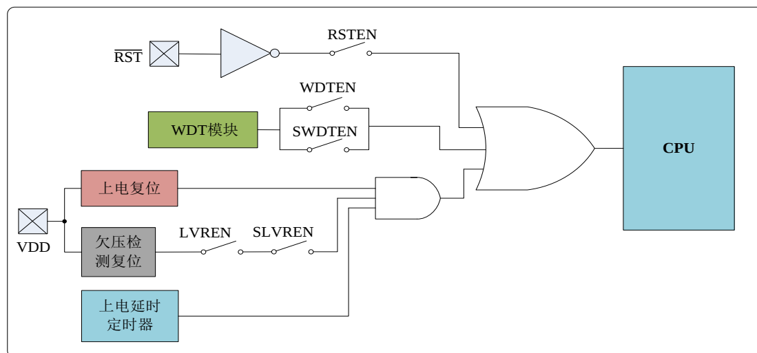
图 13.1 片内复位电路简化框图
