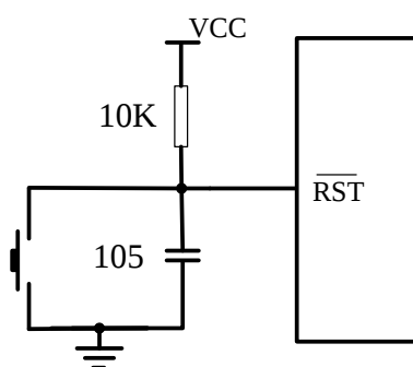
图 13.2 建议 \overline{\text{RST}} 复位电路
