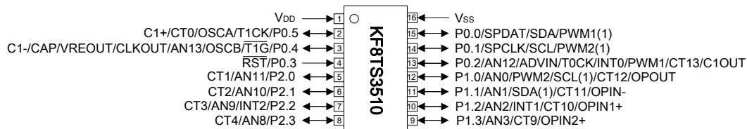
SOIC-16 引脚示意图:
