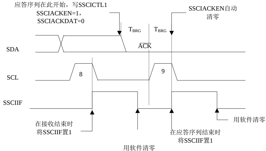
图9.17 应答序列时序波形
