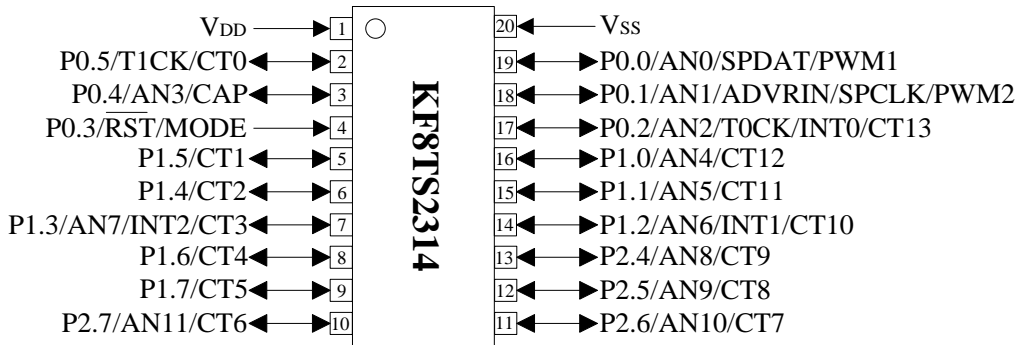
16 脚 KF8TS 2310 引脚示意图
