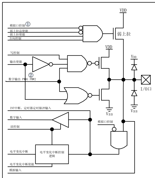
图 2.4 P0 口引脚原理框图
