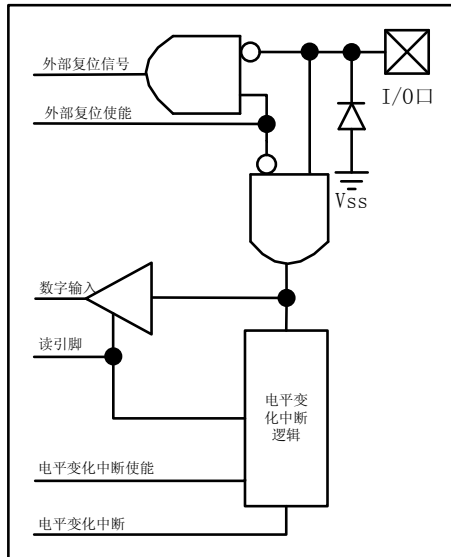
图 2.3 引脚 P0.3 原理功能框图
