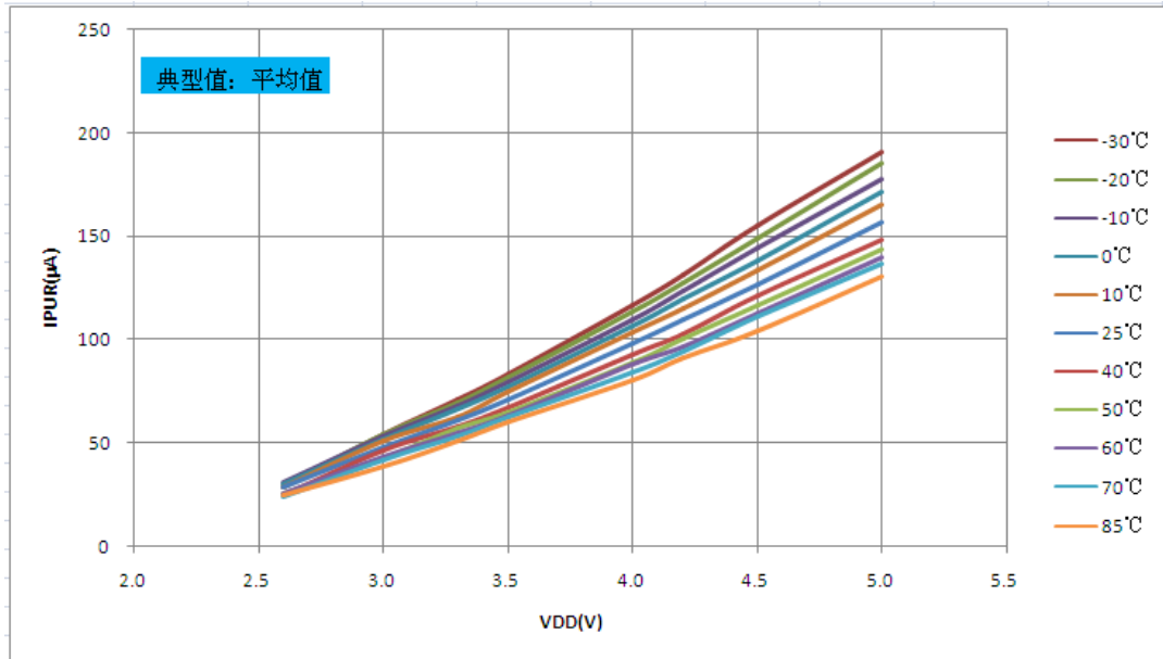
图 13-3: 弱上拉电流 I_{PUR} — VDD 关系曲线图
