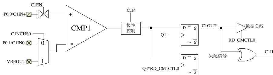
图 8-1 模拟比较器原理框图
