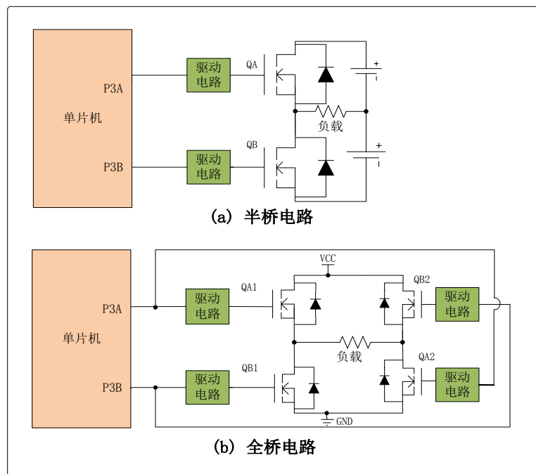
图 7-5 半桥输出模式应用举例
