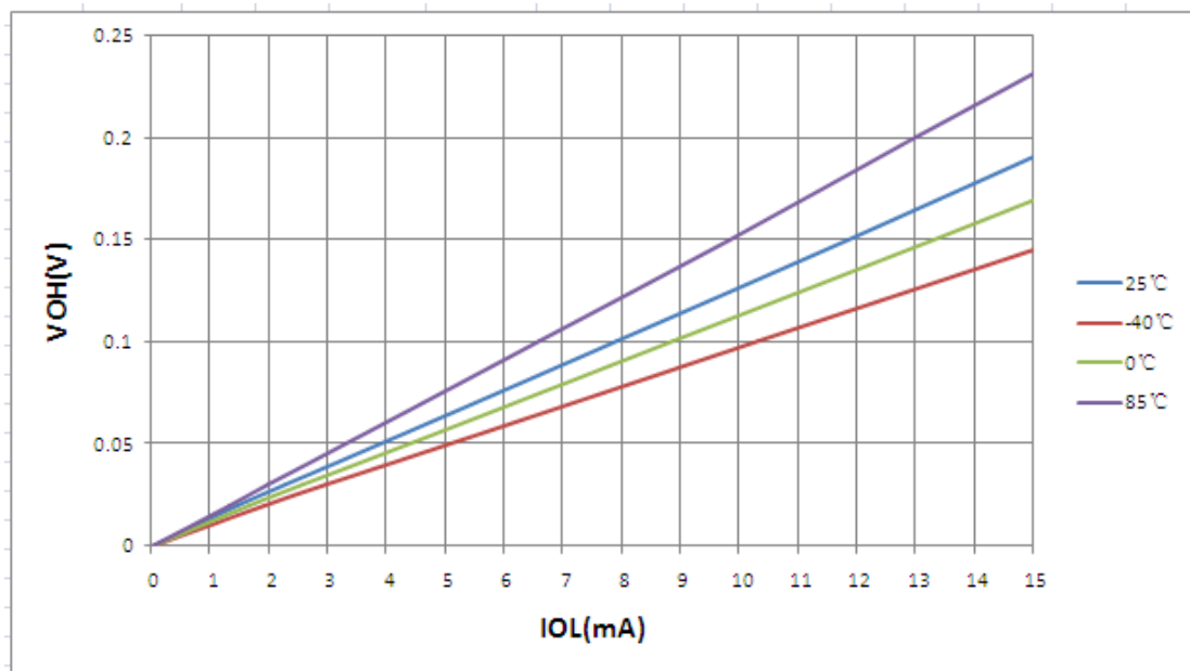
图 13-7: 不同温度时 V_{OH} - I_{OL} 关系曲线图 ( V_{DD} = 5.0V )
