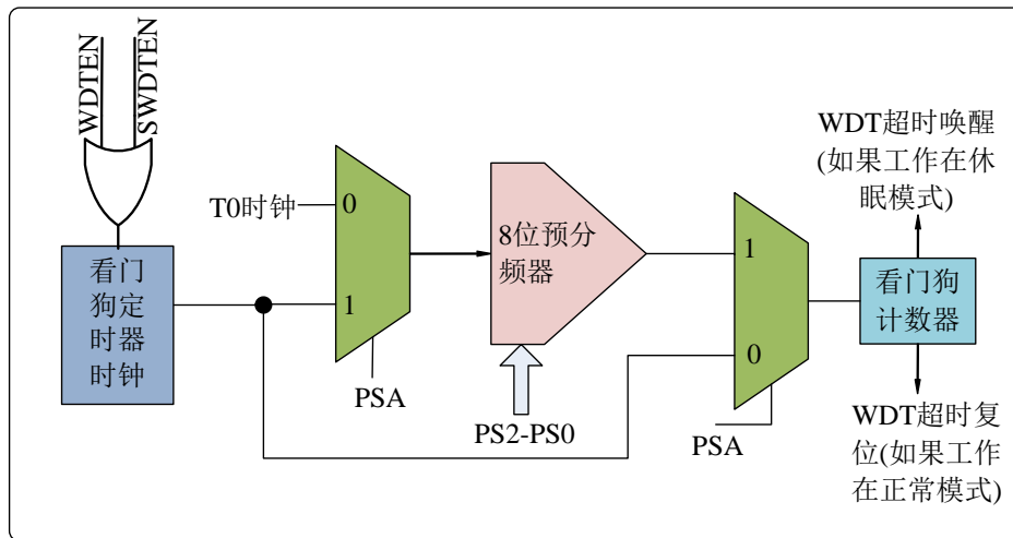
图 11-1 看门狗定时器框图
