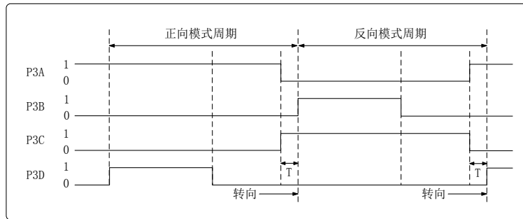
图 7-10 全桥正向、反向输出模式转换示例(高电平有效)
