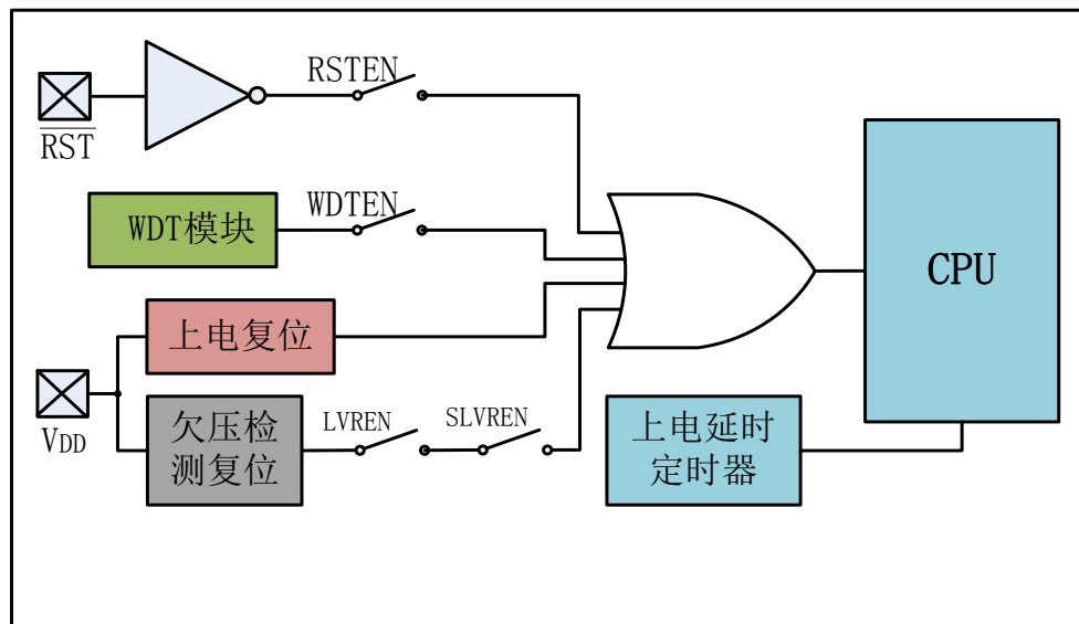
图 9-1 片内复位电路简化框图
