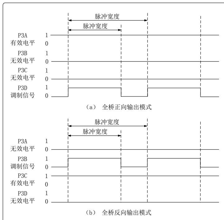
图 7-7 全桥输出模式引脚信号示例(高电平有效)
