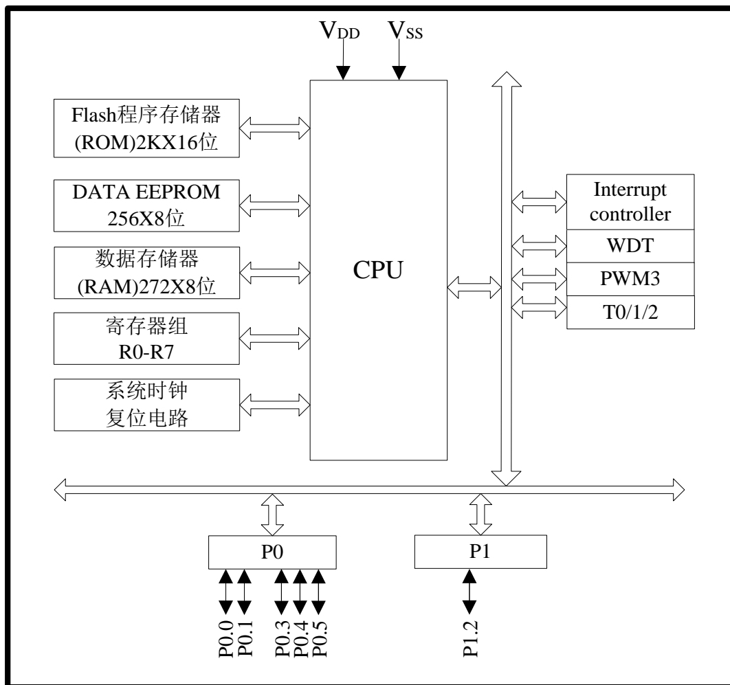
图 1-1 KF8F207 系统框图
