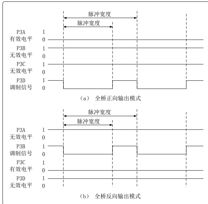
图 7-8 全桥输出模式引脚信号示例(低电平有效)
