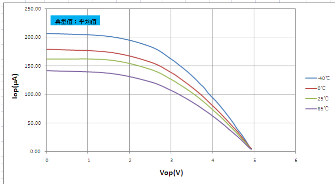
图 13-9: 上拉功能打开时端口电压 V_{OP} — 电流 I_{OP} 关系曲线图 ( V_{DD} = 5.0V )
