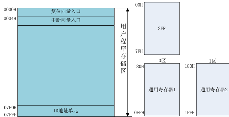
图 3-1 KF8F207 存储器组织图
