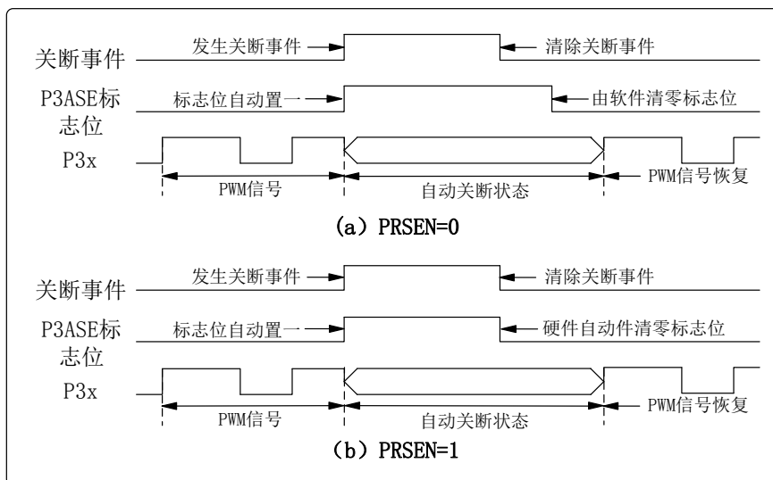
图 7-13 软件重启和自动重启 PWM 示例
