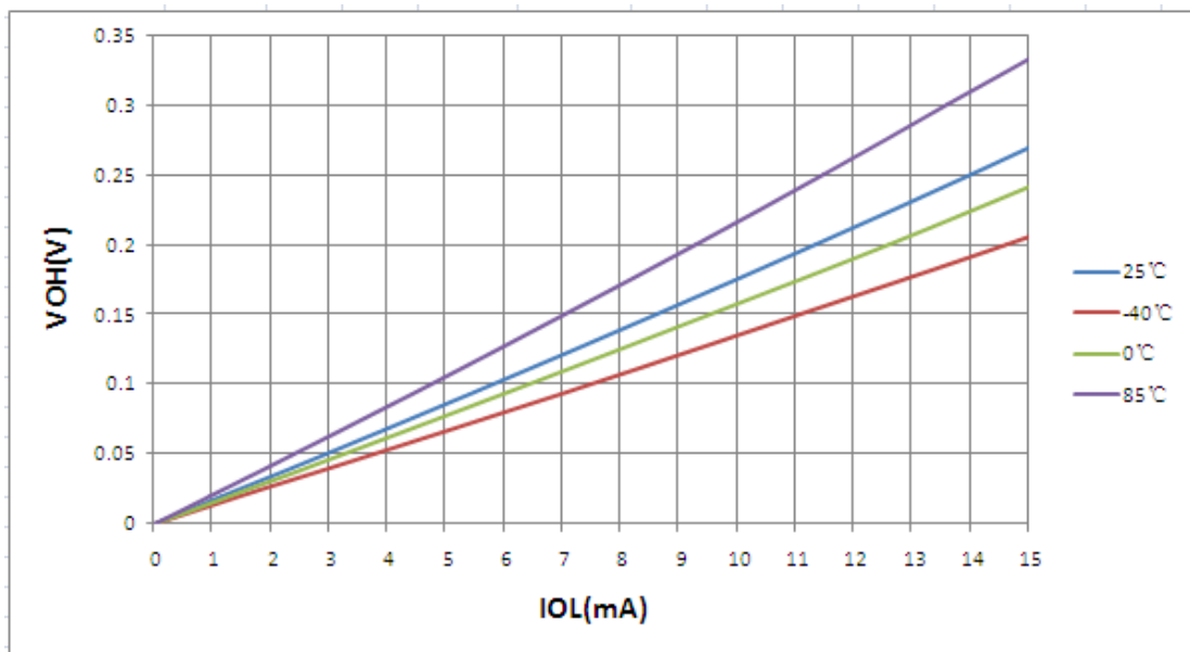
图 13-8: 不同温度时 V_{OH} - I_{OL} 关系曲线图 ( V_{DD} = 3.0V )
