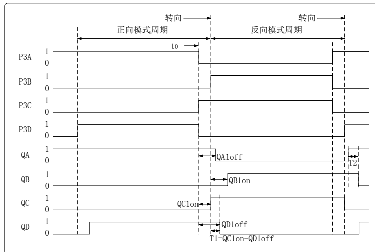
图 7-11 接近满占空比时换向时信号示例
