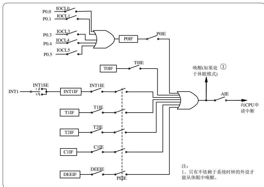
图 5-1 中断逻辑
