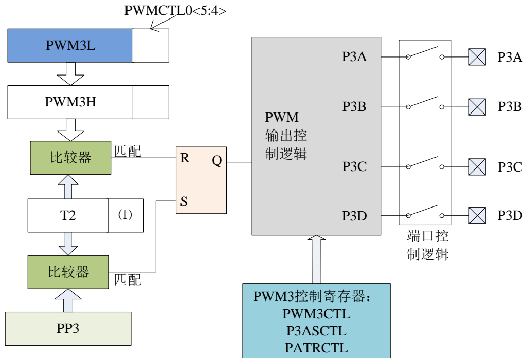
7-1 PWM3 原理框图
