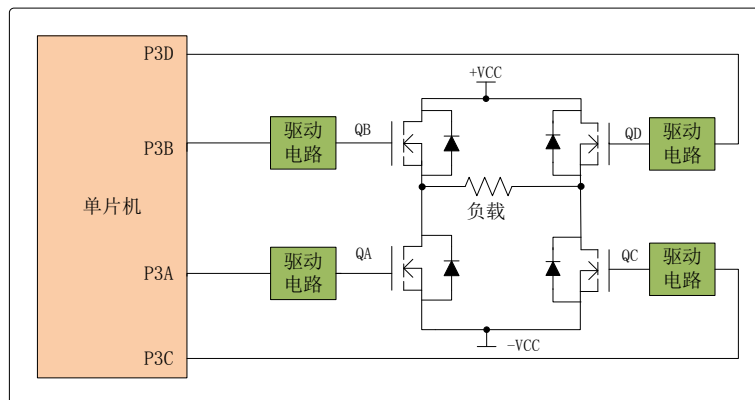
图 7-9 全桥输出模式应用电路示例
