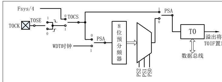
图 6-1 预分频器框图
