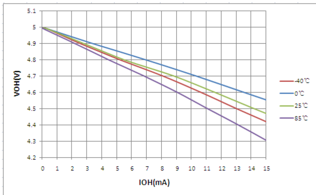
图 13-5: 不同温度时 V_{OH} - I_{OH} 关系曲线图 ( V_{DD} = 5.0V )
