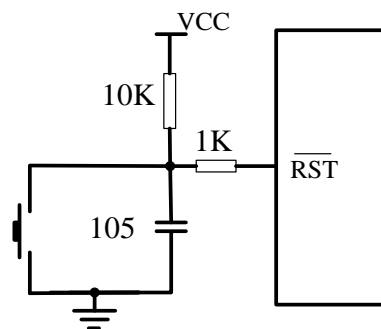
图 9-2 建议 \overline{\text{RST}} 复位电路
