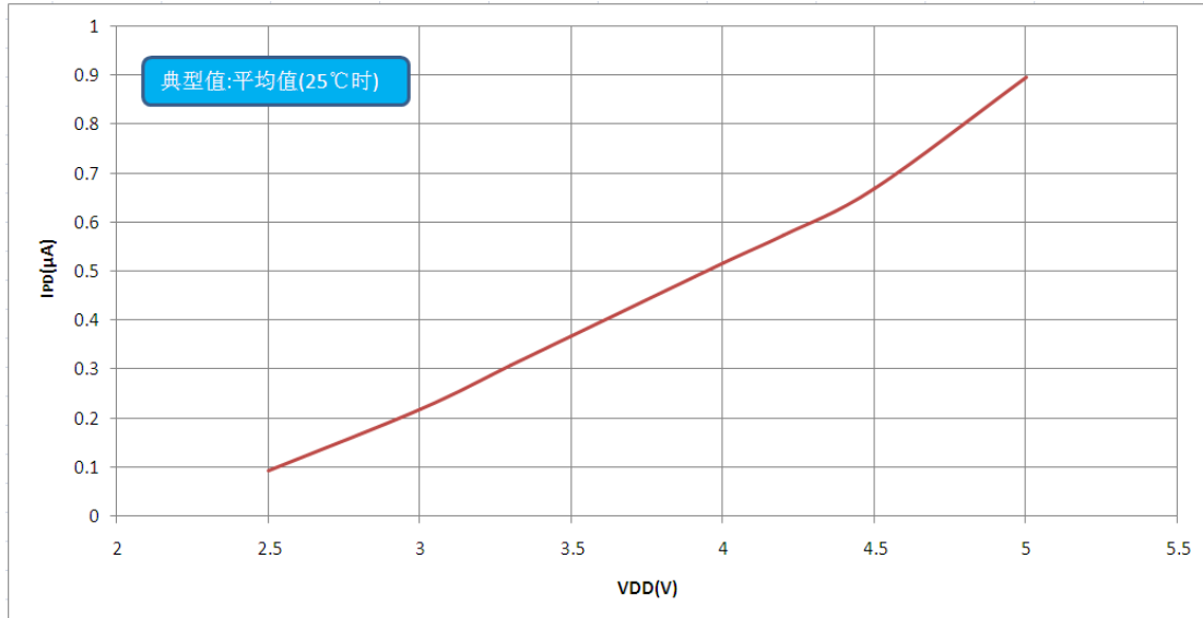
图 13-2: 不同 VDD 时典型 I_{DD} — VDD 关系曲线图
