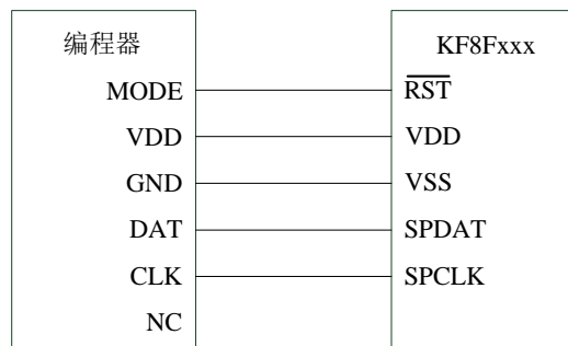
图 1-7 KF8F207 在线串行编程连接图
