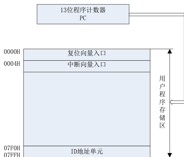
图 3-3 KF8F207 程序存储器映射
