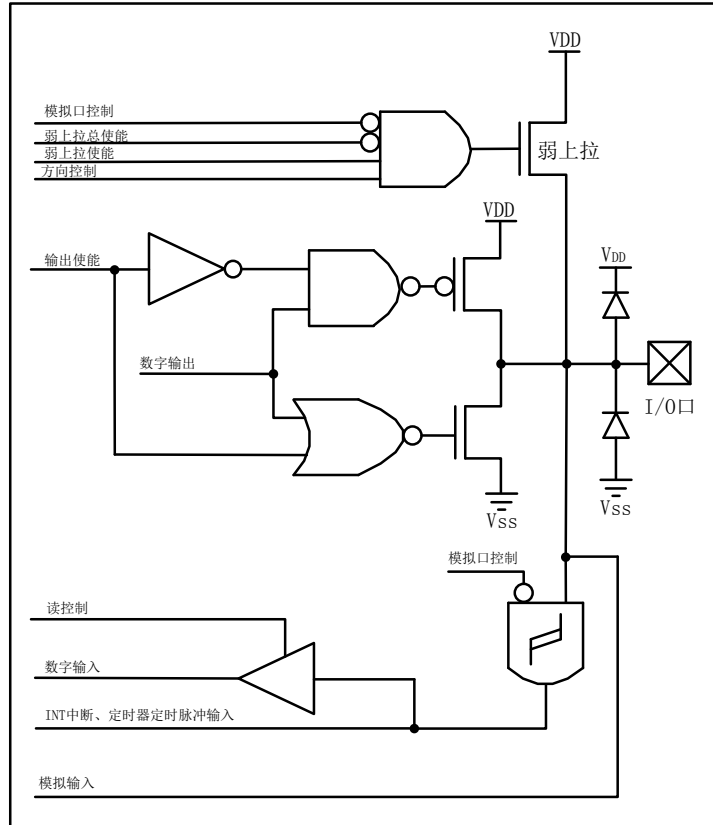
图 2-3 P1.2 口引脚原理功能框图
