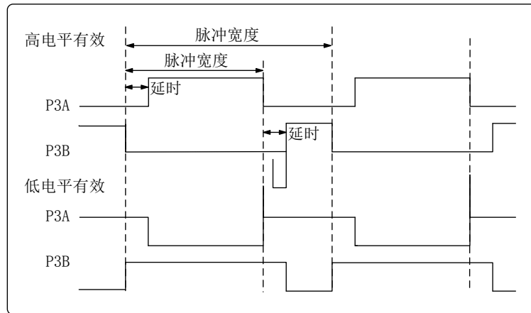
图 7-4 半桥输出模式输出信号示例
