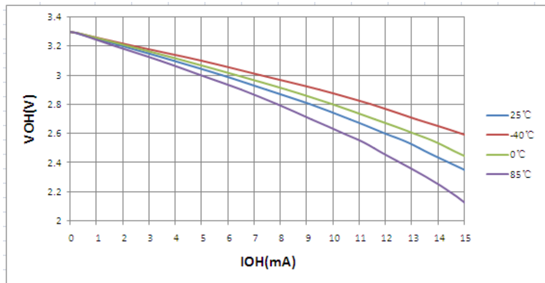
图 13-6: 不同温度时 V_{OH} - I_{OH} 关系曲线图 ( V_{DD} = 3.0V )
