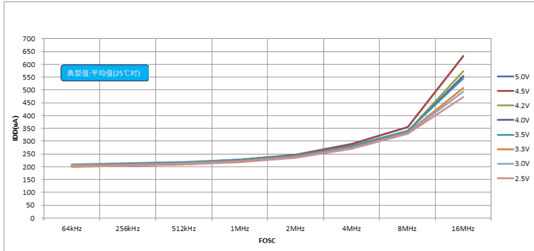
图 13-1: 不同 VDD 时典型 I_{DD} — FOSC 关系曲线图
