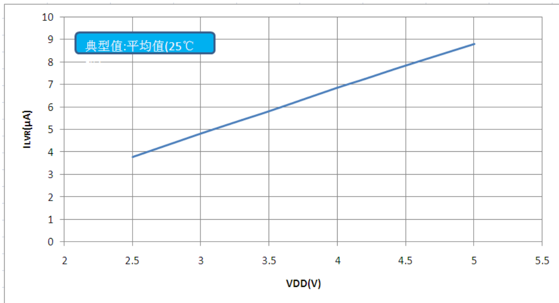
图 13-4: 欠压复位电流 I_{LVR} — VDD 关系曲线图
