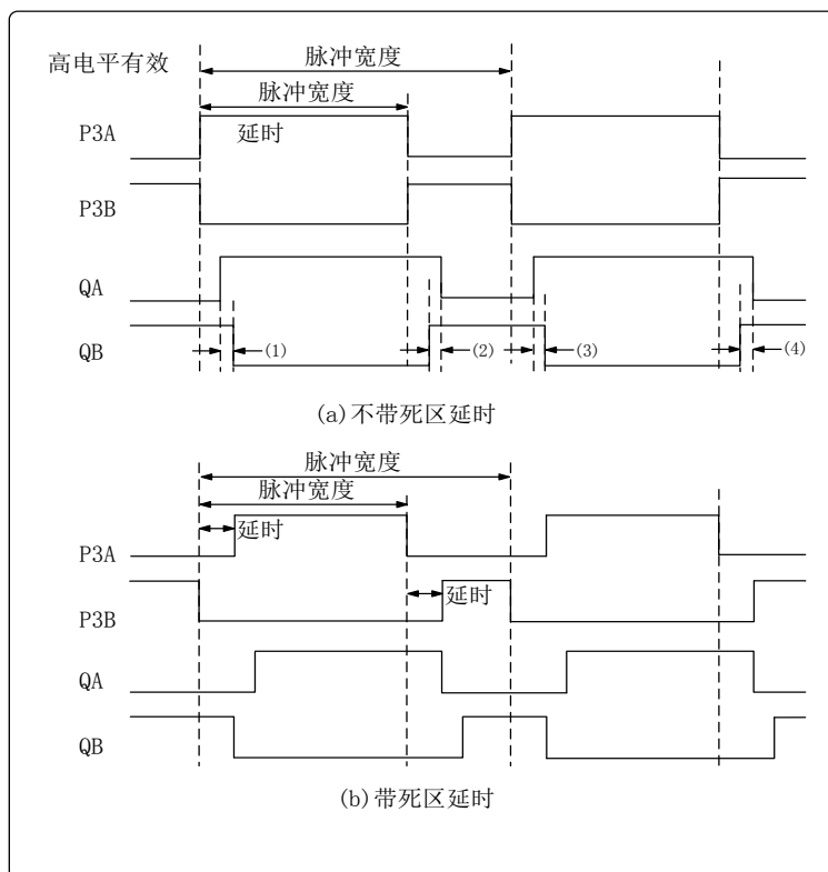
图 7-6 带死区控制和不带死区控制时的信号示例
