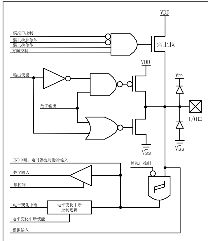
图 2-2 引脚 P0.0~P0.1、P0.4、P0.5 原理功能框图
