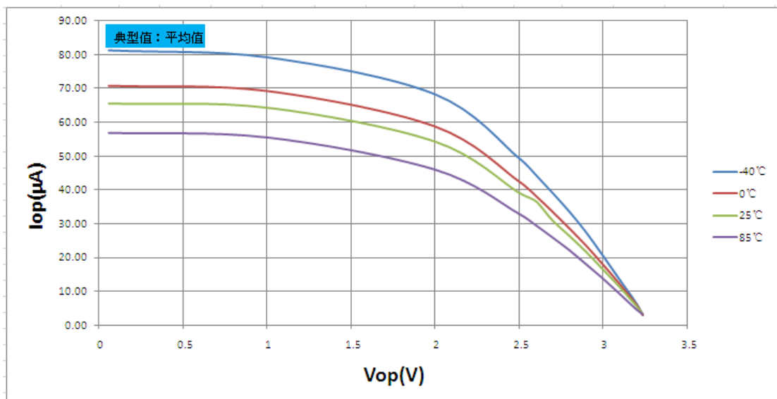
图 13-10: 上拉功能打开时端口电压 V_{OP} — 电流 I_{OP} 关系曲线图 ( V_{DD} = 2.7V )
