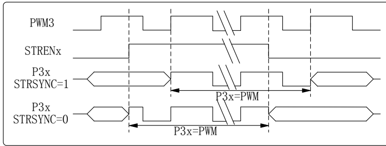
图 7-3 单输出模式 PWM 输出引脚切换
