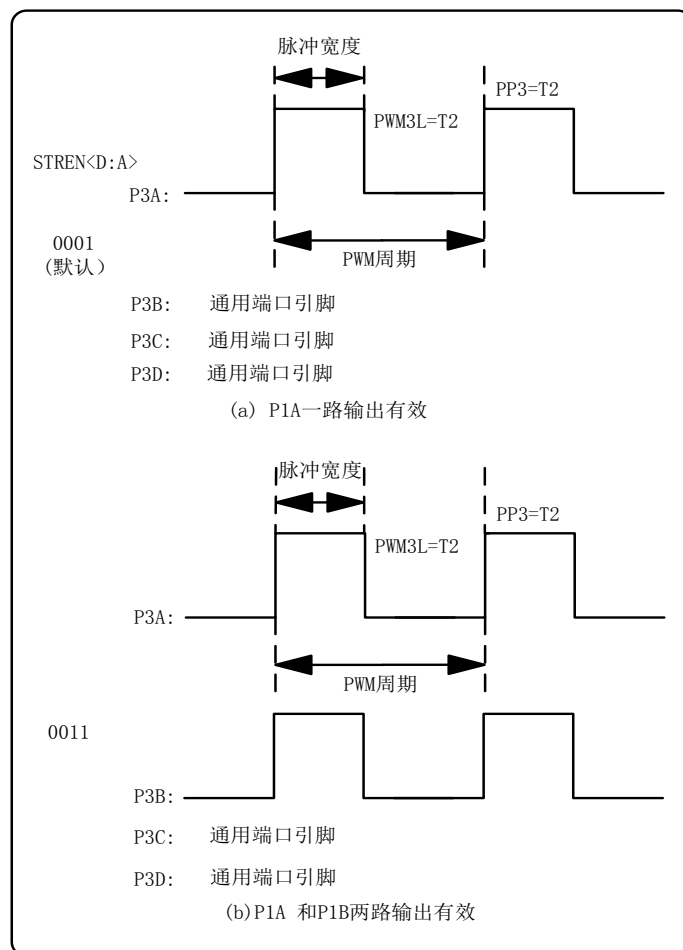
图 7-2 PWM3 的输出示例
