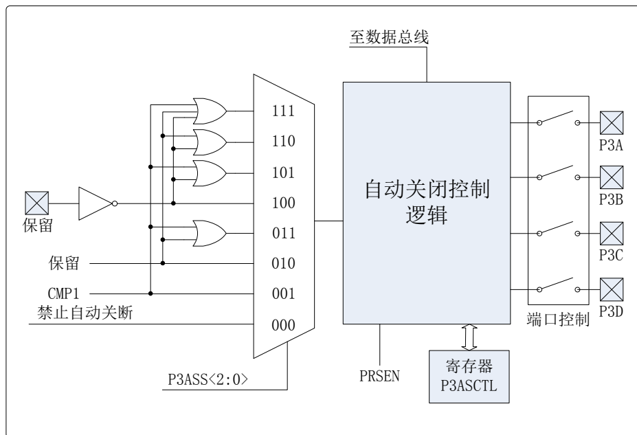
图 7-12 自动关断模式原理框图
